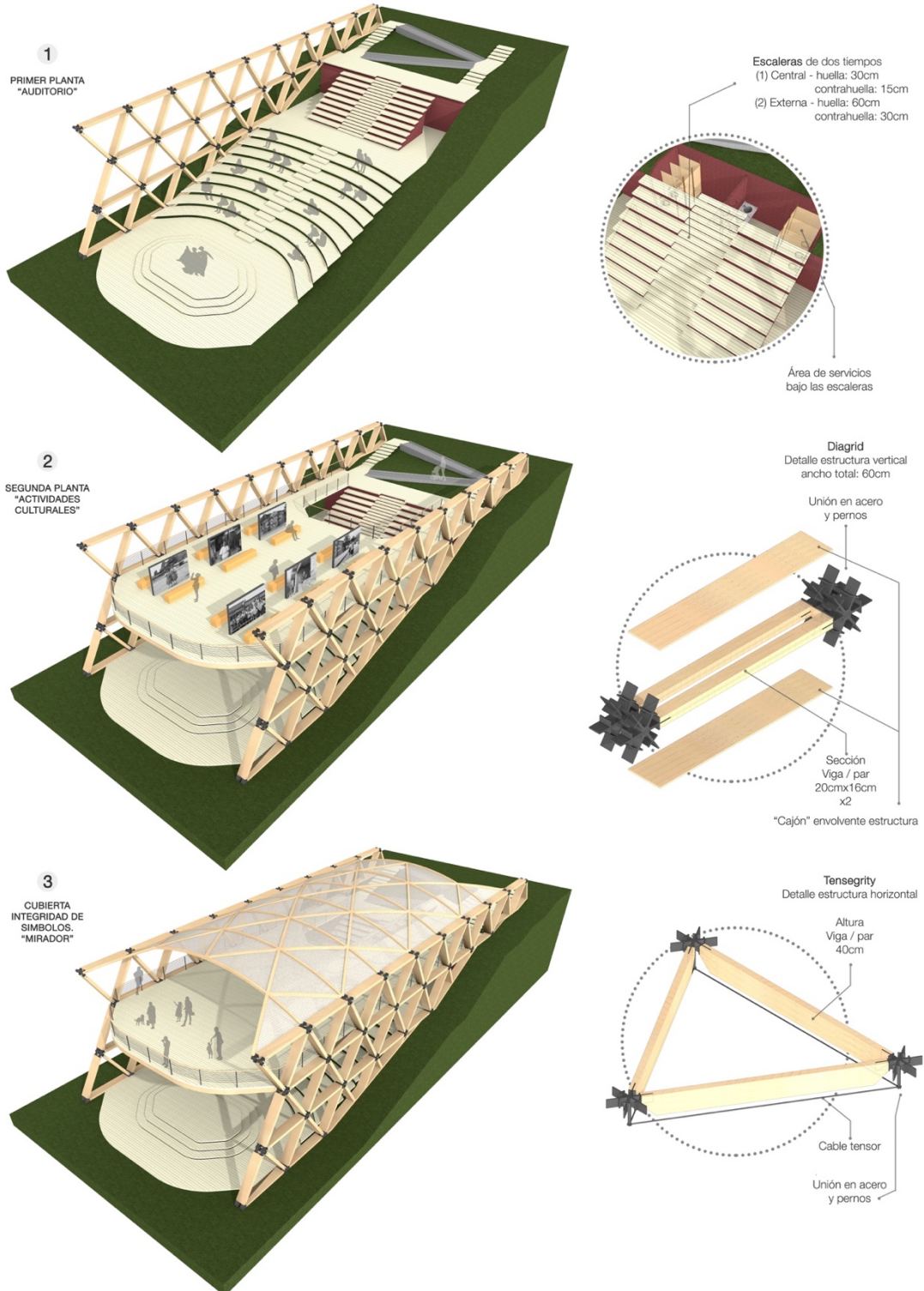
Ilustración 38: Casa cultural (niveles y desarrollo constructivo)
