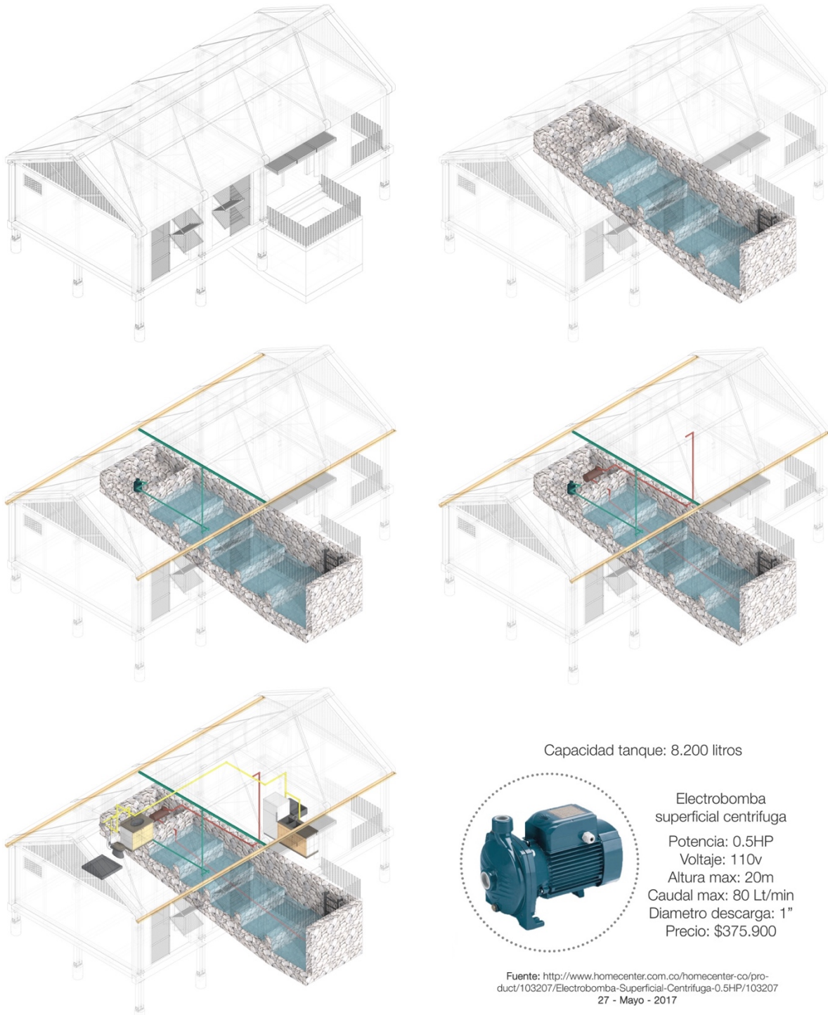
Ilustración 34: Recolección de aguas lluvias
