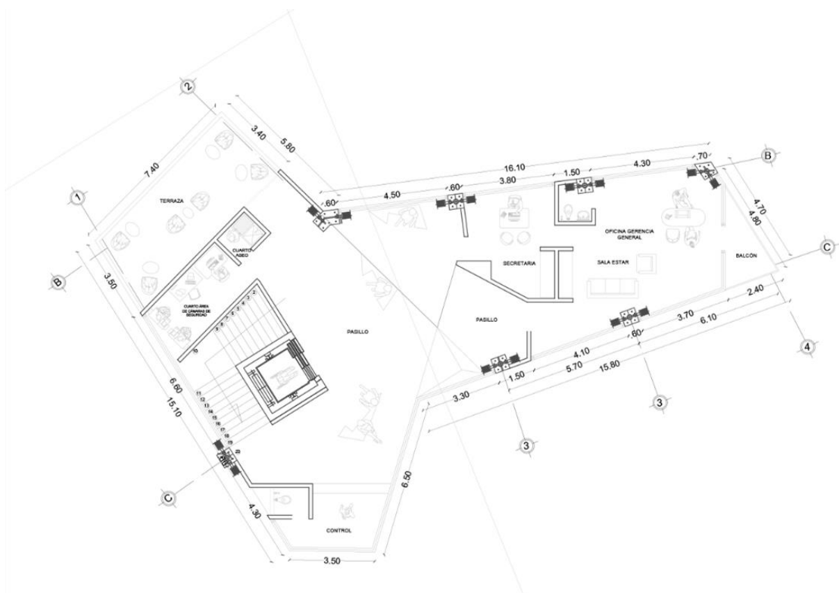
Imagen 33. Quinta planta
