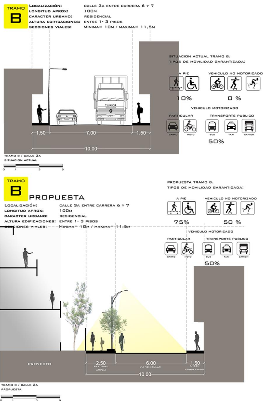
Imagen 16. Perfil sector B
