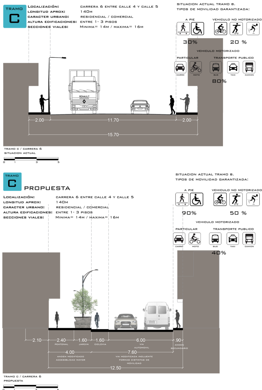
Imagen 18. Perfil sector C
