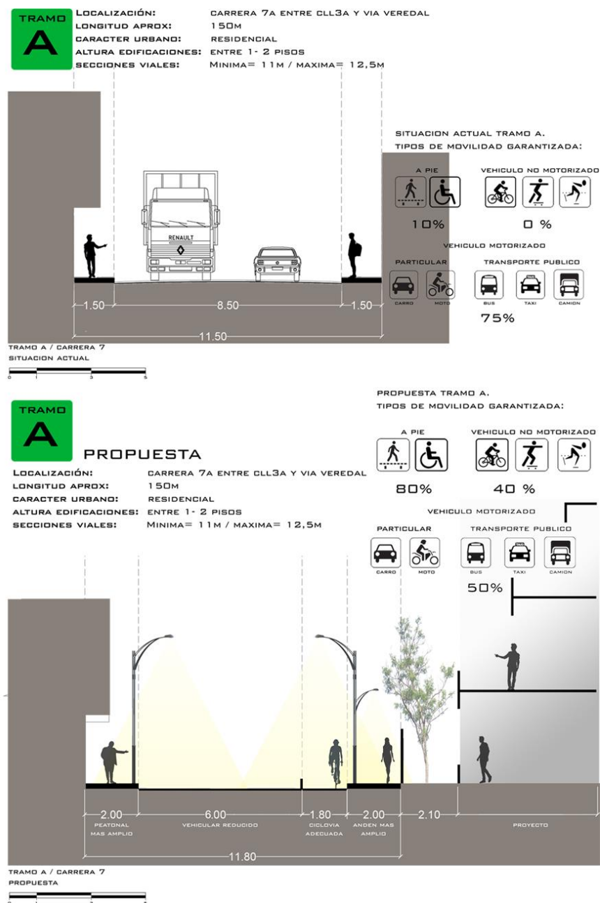
Imagen 15. Perfil sector A
