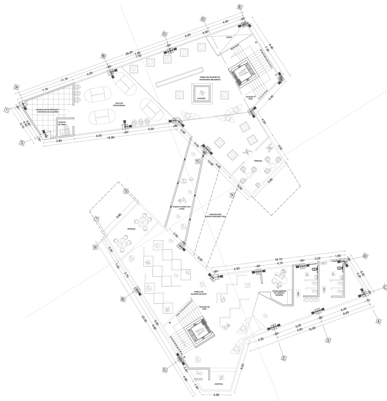
Imagen 31. Tercera planta
