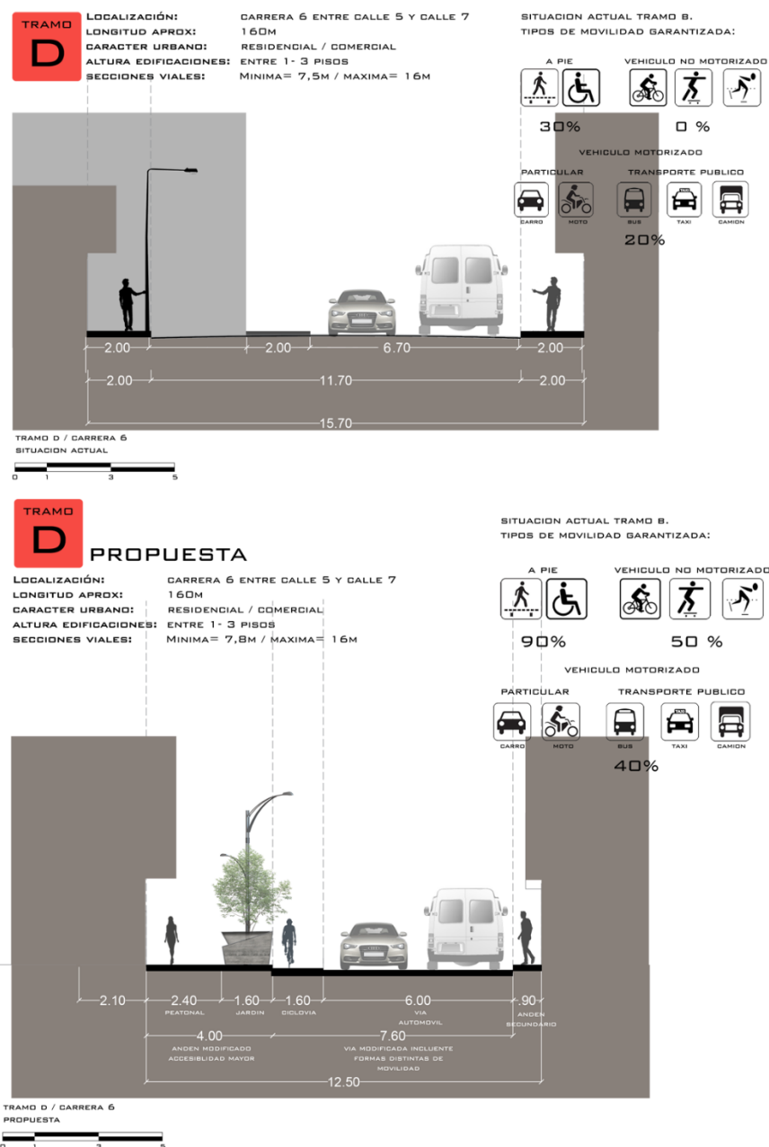
Imagen 19. Perfil sector D
