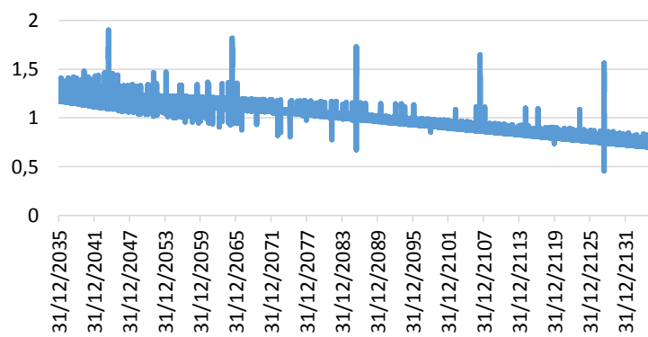
Comportamiento serie sintética de caudales RCP 8.5
