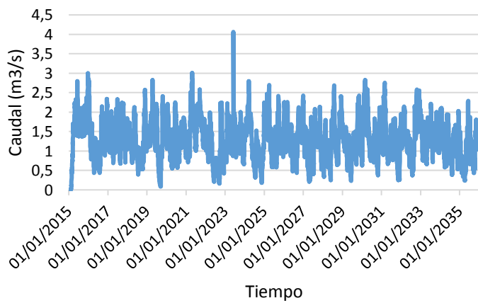
Caudales bajo el escenario RCP 8.5
