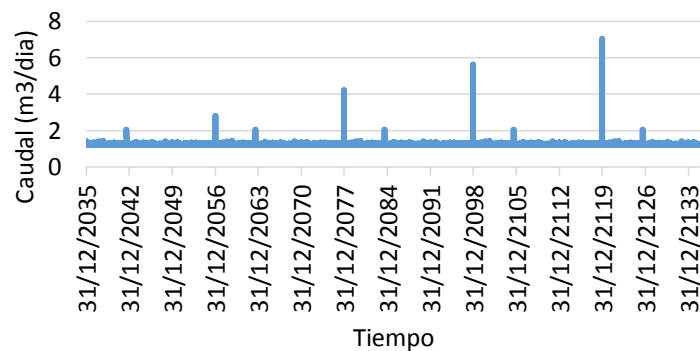
Comportamiento de la serie sintetica de caudal RCP 4.5
