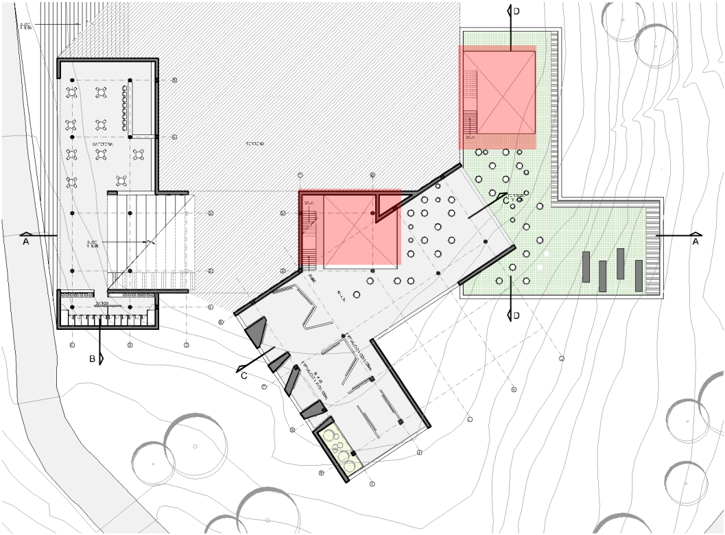
PLANTA N -5.05 ESCALA GRÁFICA
