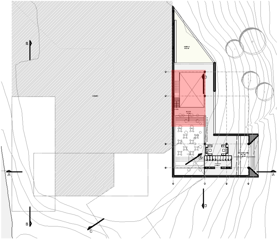
PLANTA N -9.05 ESCALA GRÁFICA
