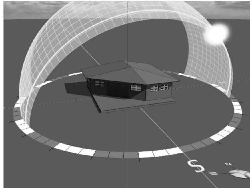
Figura 20. Heliodón
