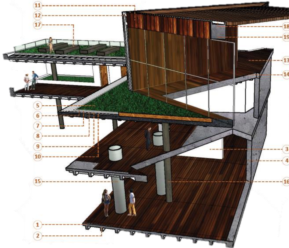
Figura 44. Sección fugada
