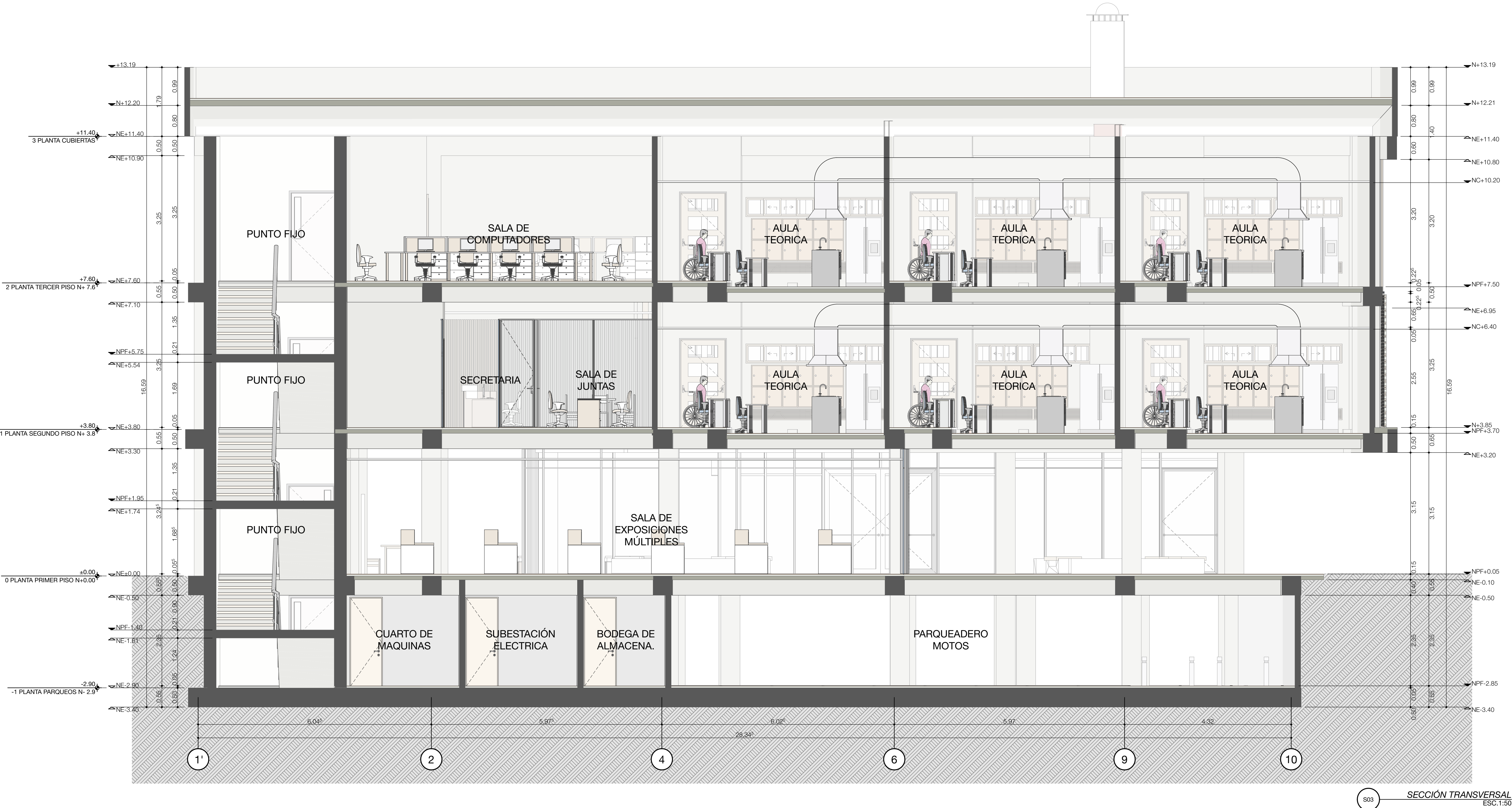
S03 SECCIÓN TRANSVERSAL ESC.1:50
