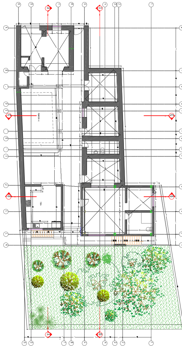
Planta Primer Piso
