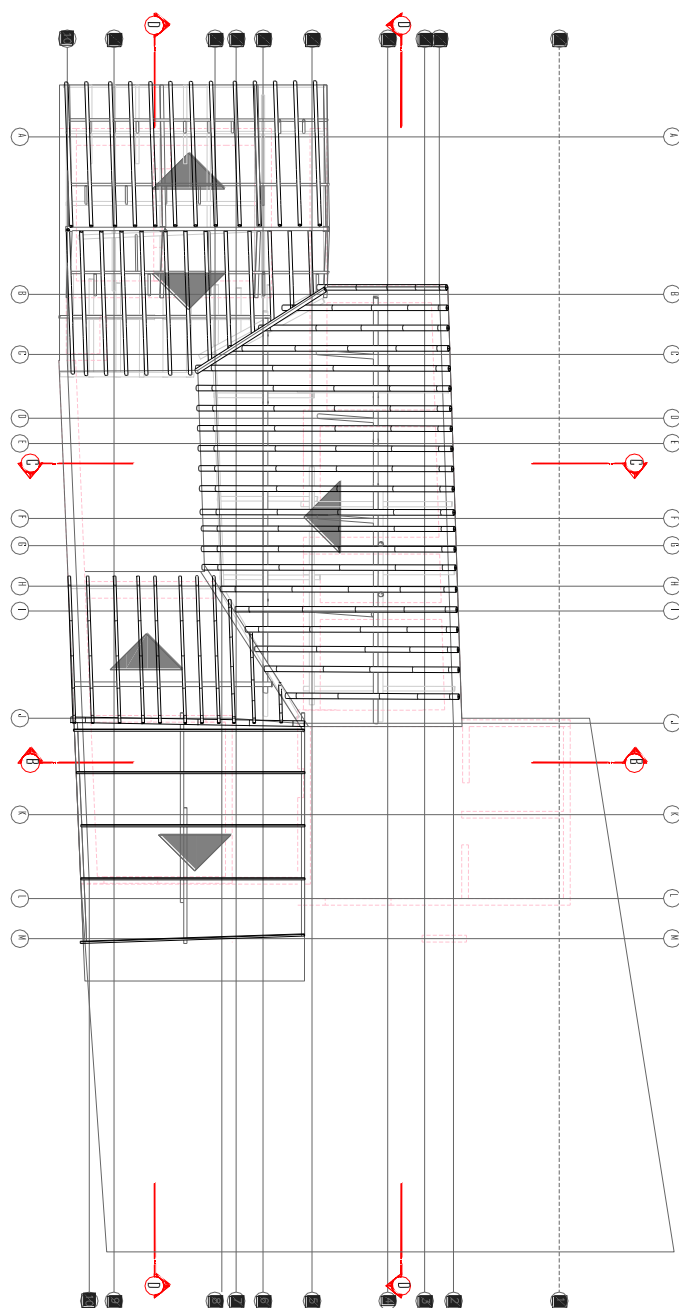
Planta Estructural De Cubierta
