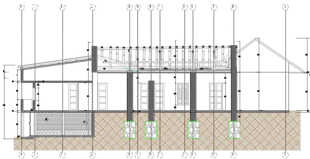
Corte A-A
