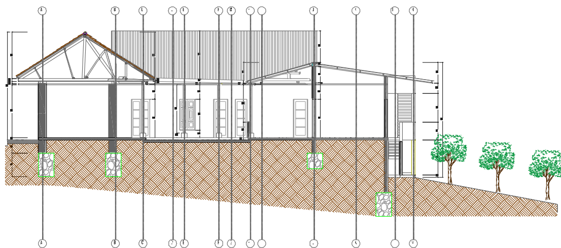
Corte D-D
