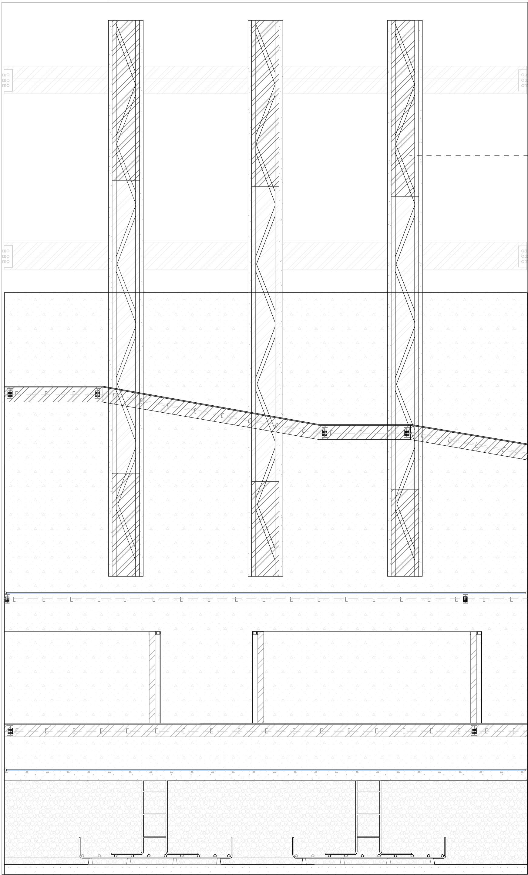
SECCION LONGITUDINAL ESC: 1:50
