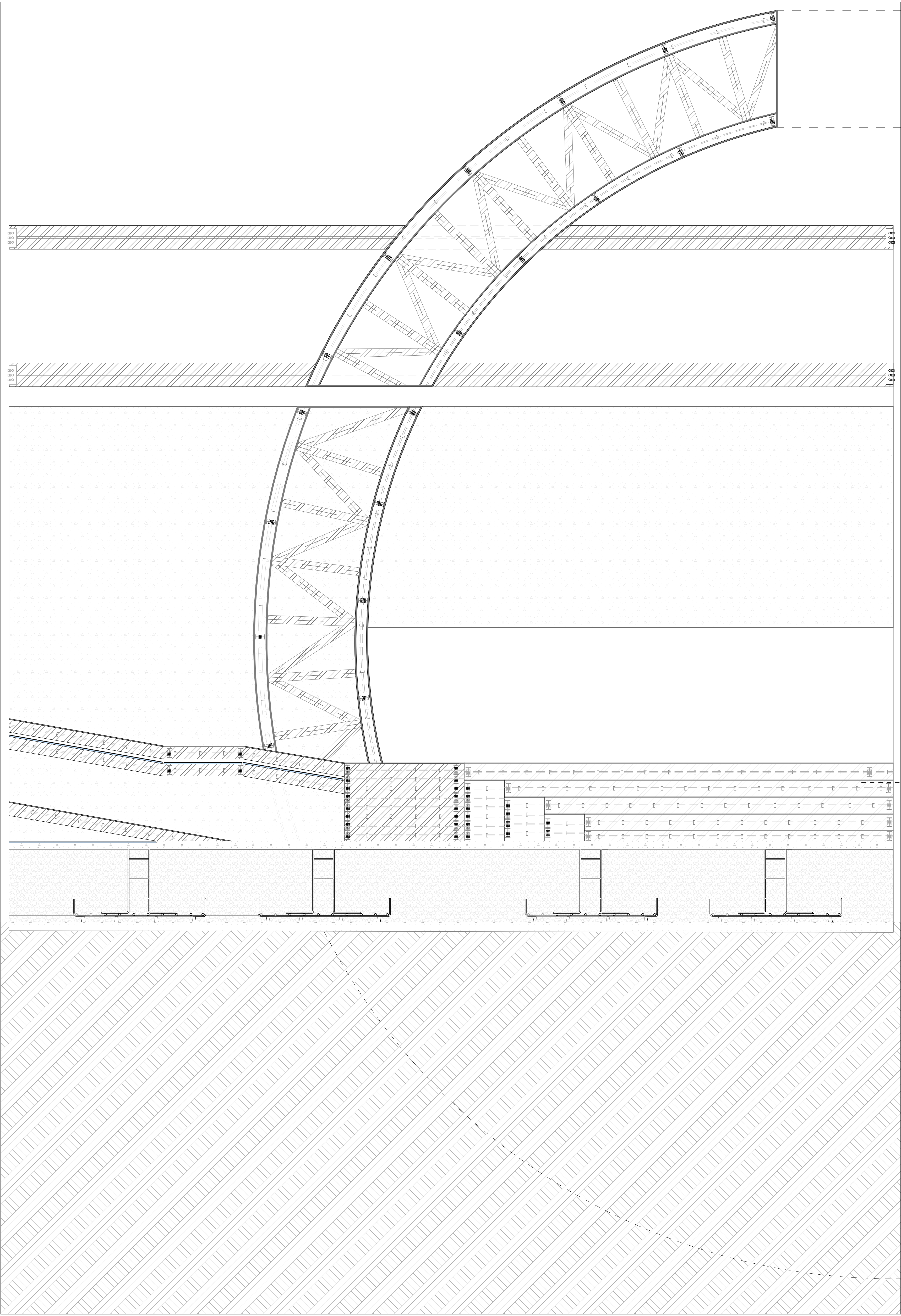
SECCION LONGITUDINAL ESC: 1:50
