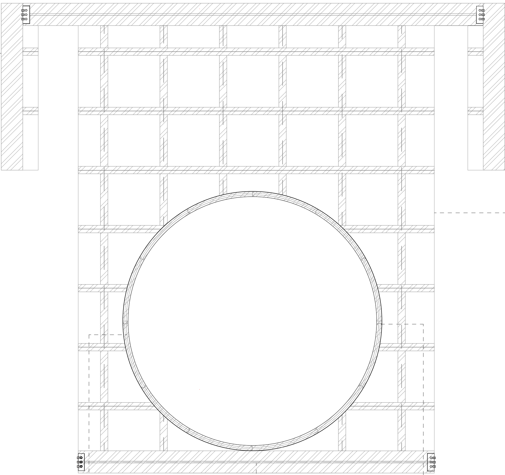
DETALLE CONSTRUCTIVO PANEL FLOTANTE ESC: 1:50
