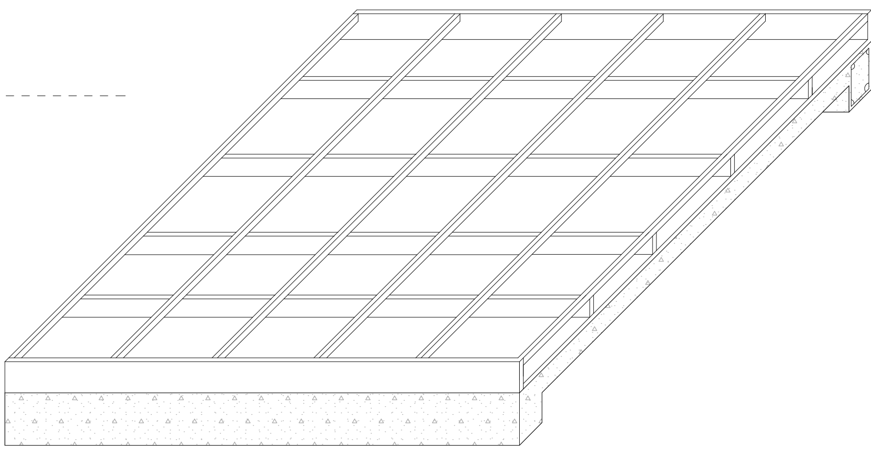
DETALLE CONSTRUCTIVO PLACA DE HORMIGON CON PERFILES STEEL FRAMING ESC: 1:50
