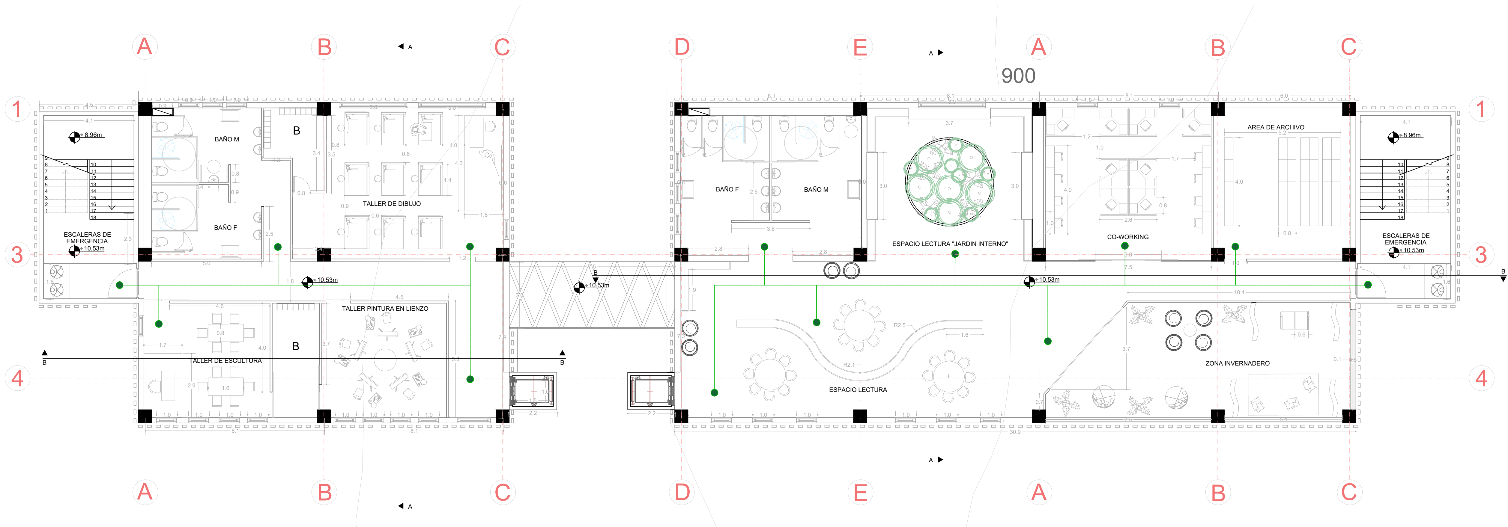
A19 PLANTA TALLER Y BIBLIOTECA TERCER PISO ESC 1:150
