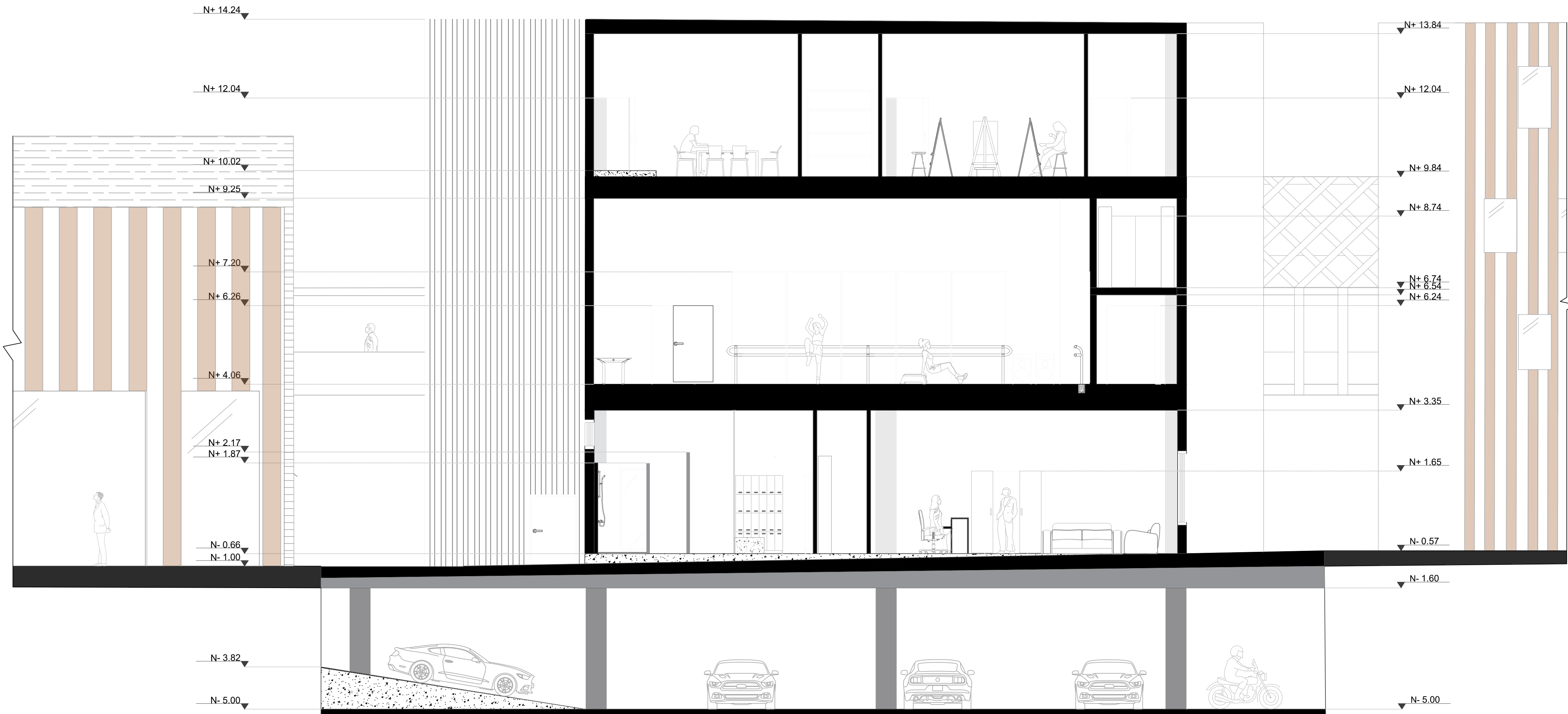
A20 CORTE LONGITUDINAL BB ESC 1:70
