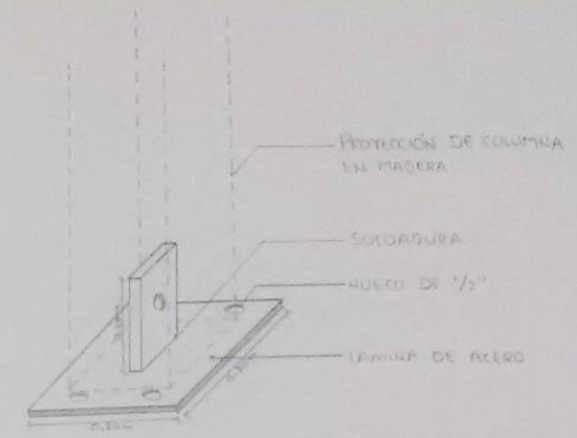
DETALLE PLATINA EN ACERO ESC 1:10
