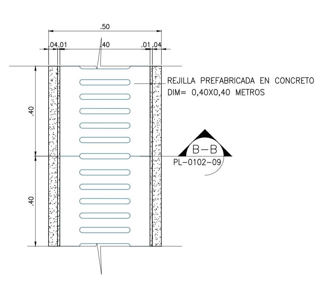
4 DETALLE CARCAMO ESC. 1:10
