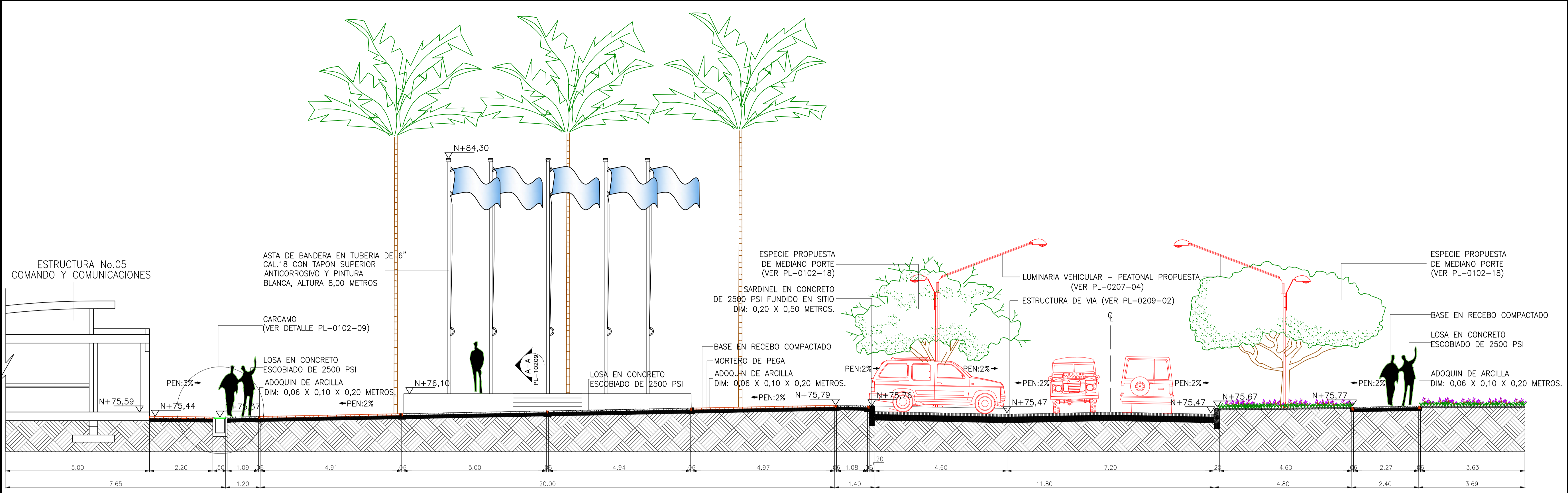
2 CORTE 4-4 ESC. 1:75
