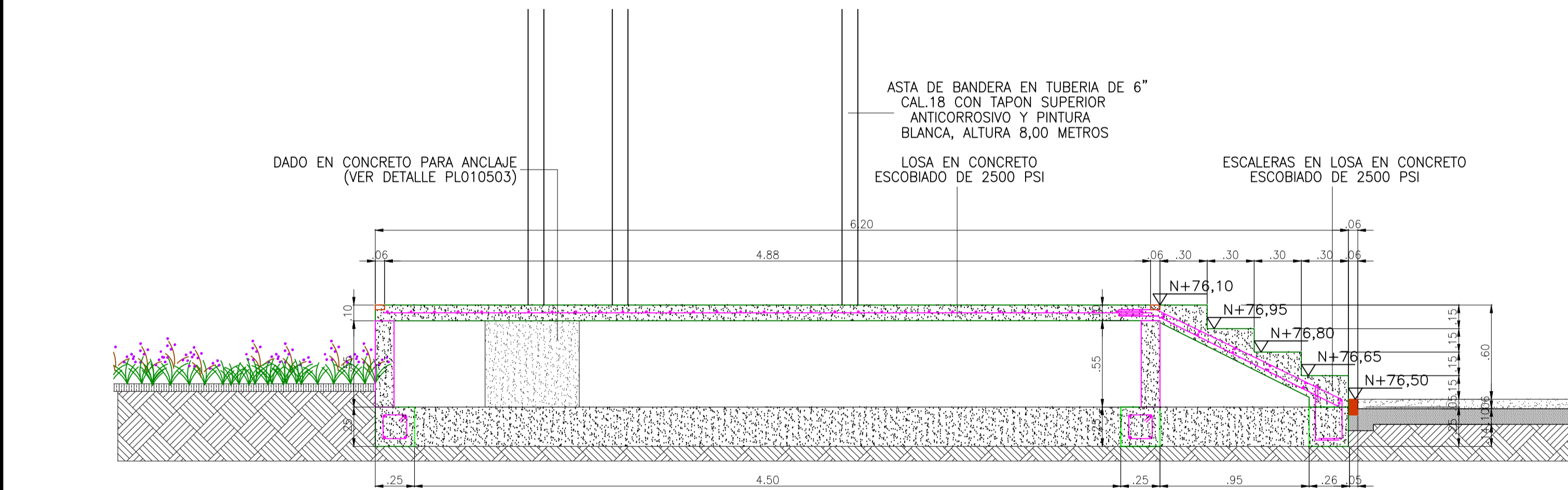
3 CORTE A-A ESC. 1:25
