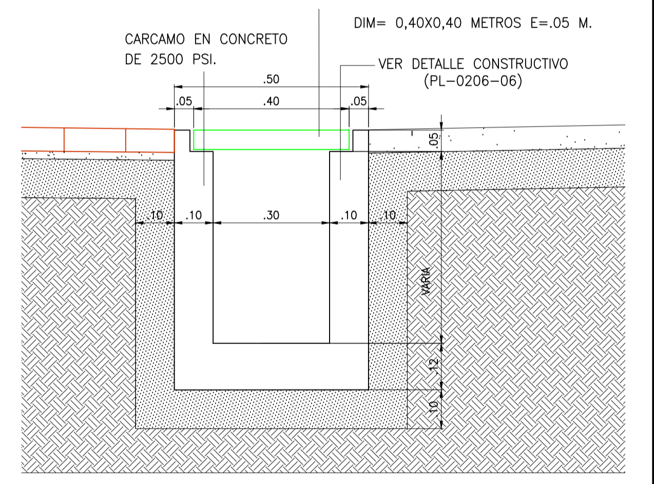
5 CORTE B-B ESC. 1:10
