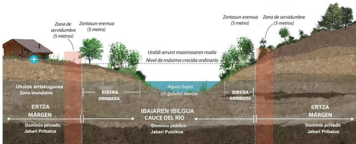
Figura 57. Esquema general de las componentes de un río con sus reguladores hidrológicos naturales.
