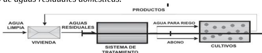
Figura 55. Esquema general de un sistema descentralizado integrado y sostenible para el tratamiento de aguas residuales domésticas.
