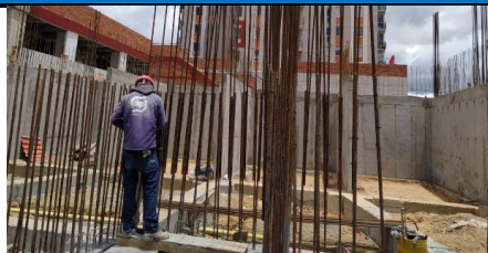
#73 Amarre de refuerzo en muros
