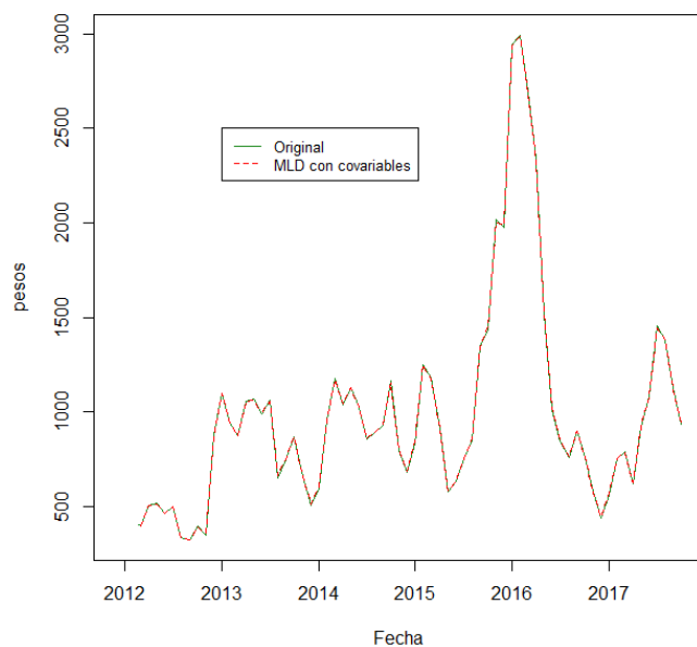
Figura 8: Estimación del precio por MLD con covariables
