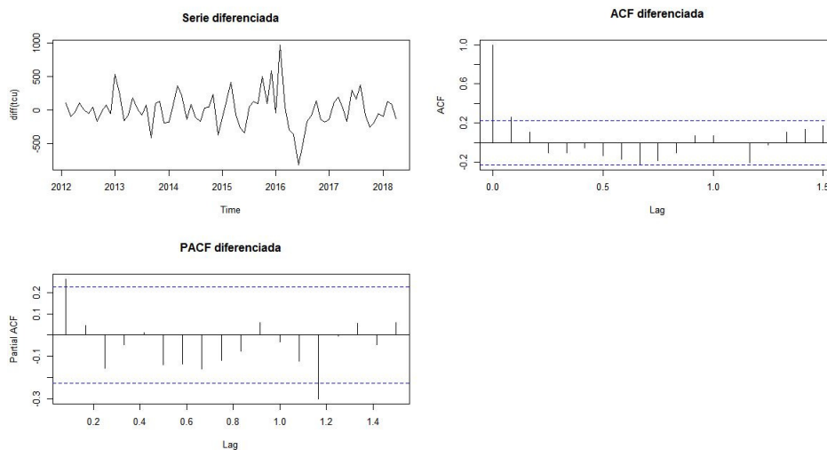
Figura 3: ACF y PACF para la serie diferenciada
