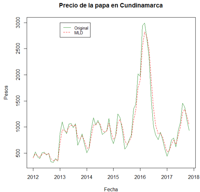
Figura 5: Estimación del precio por MLD
