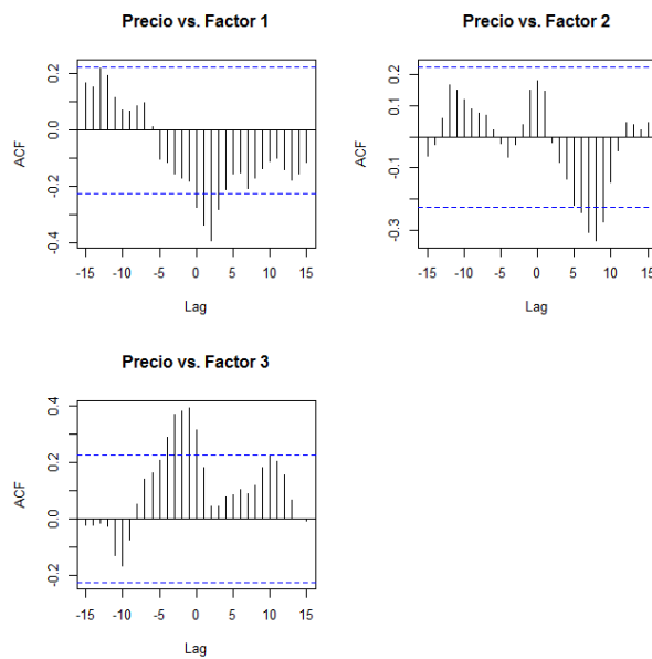
Figura 7: ACF del precio teniendo en cuenta los factores
