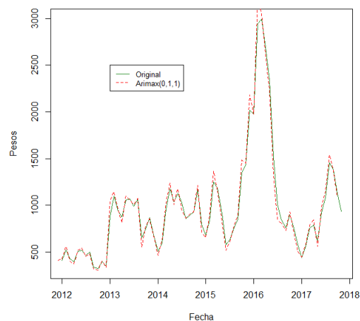
Figura 6: Estimación del precio por ARIMAX
