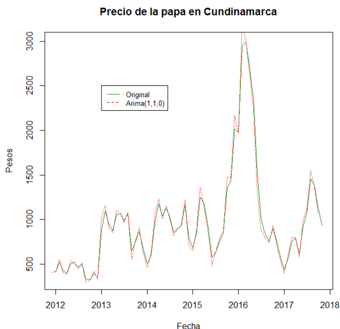
Figura 4: Estimación del precio por ARIMA
