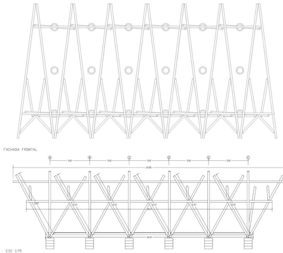
Figura 18. Planta y fachada frontal de la Casa Comunal Renacer de Chamanga.
