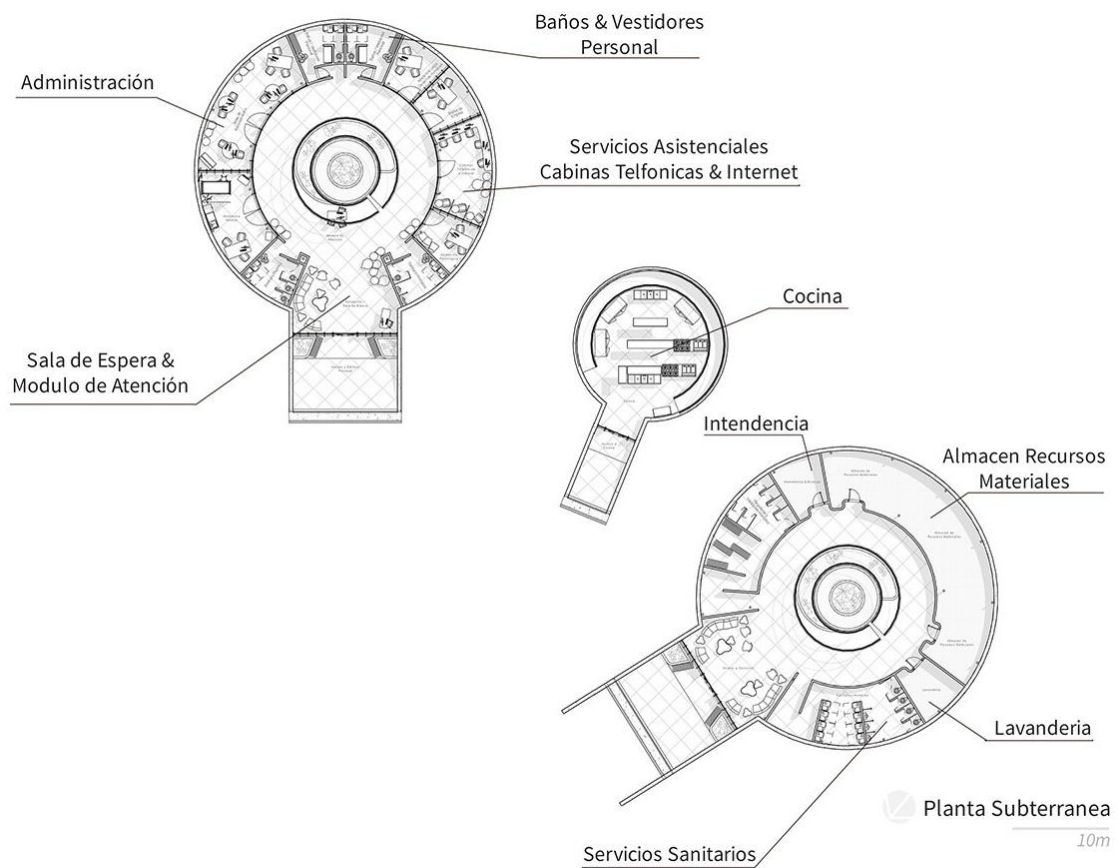
Figura 10. Plantas generales del Centro de Atención al Migrante
