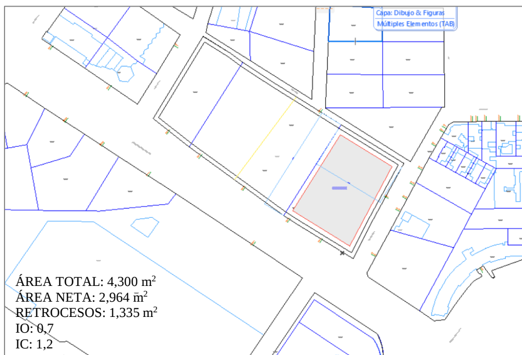
Figura 35. Planimetría del lote y su entorno inmediato
