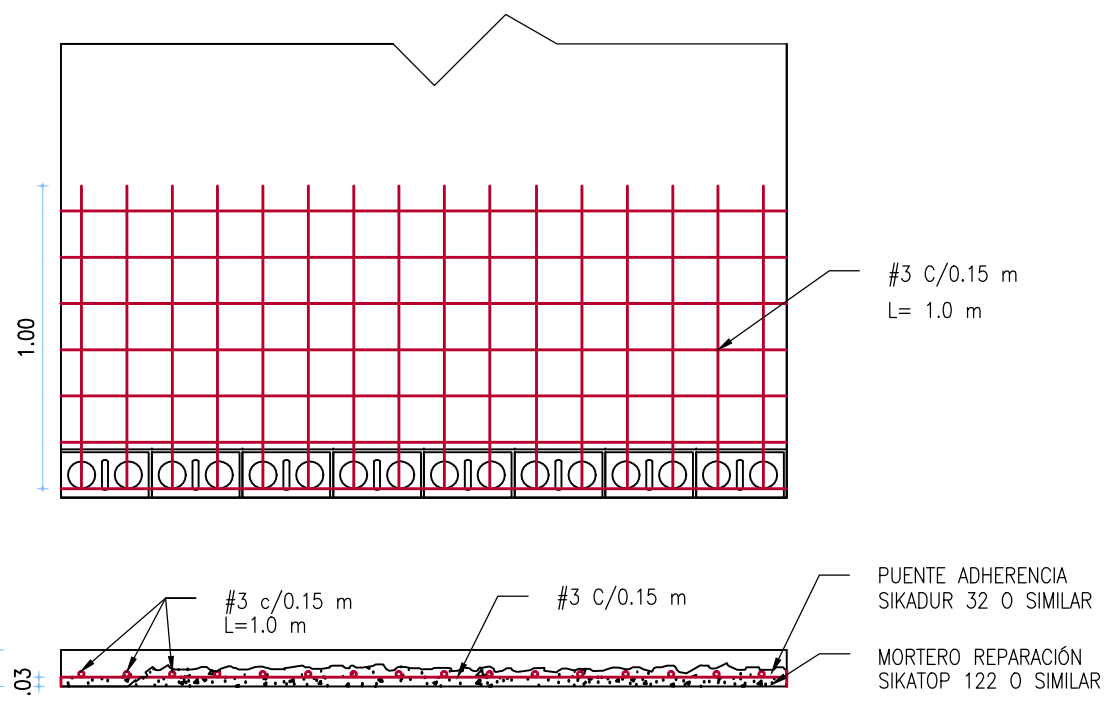
DETALLE INTERVENCIÓN PLACA ENTREPISO ESC 1 :25
