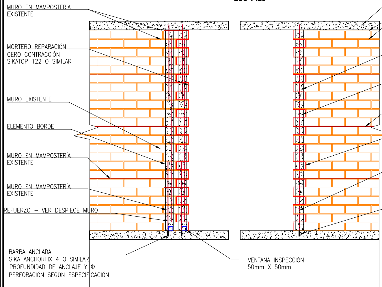
DETALLE INTERVENCIÓN # 3 ESC 1 :25
