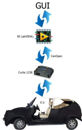
Fig. 6. Flujo de información entre el diseño eléctrico y mecánico.
