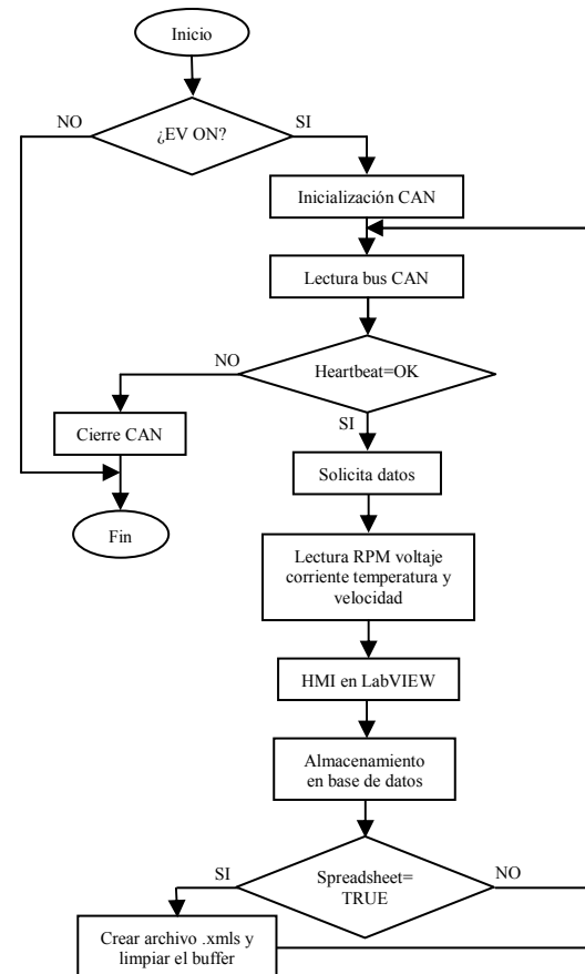
Fig. 3. Diagrama de flujo del algoritmo implementado.
