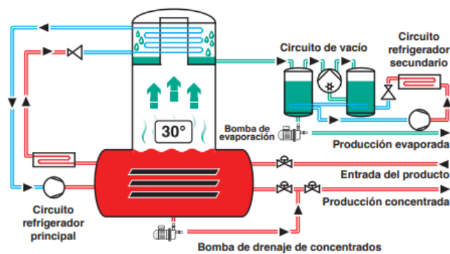
Esquema de funcionamiento evaporadores al vacío a bomba de calor MONO EFECTO
