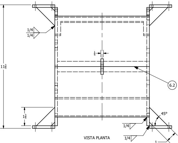
VISTA PLANTA
