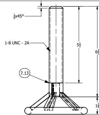
VISTA PLANTA
