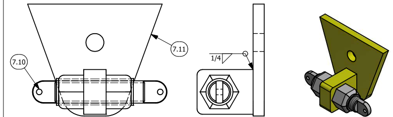
VISTA FRONTAL ESCALA 1 : 1
