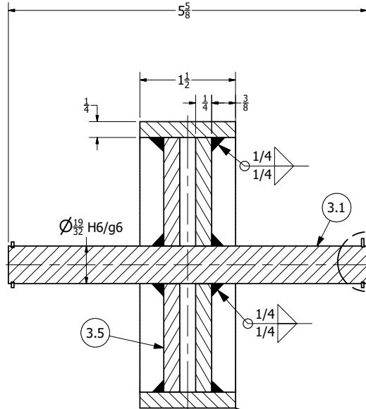
SECTION W-W SCALE 1 : 1
