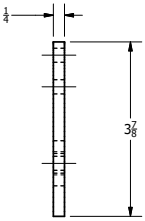
VISTA LATERAL
