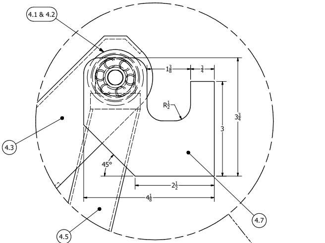
DETAIL Y SCALE 1:1
