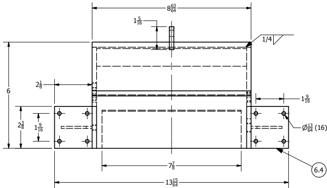
VISTA FRONTAL ESCALA 1 : 2.5
