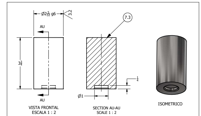
ISOMETRICO
