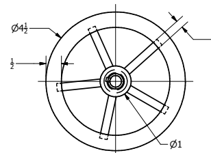
VISTA FRONTAL ESCALA 1 : 2
