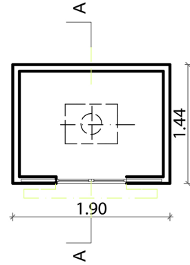
PLANTA ESC 1:50
