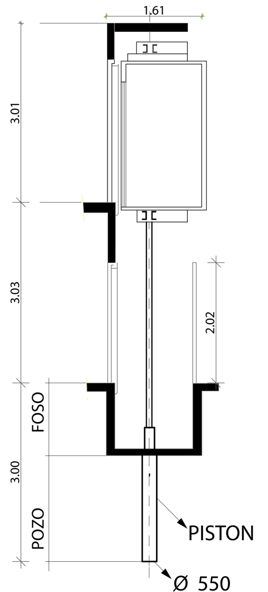
SECCION A-A' ESC 1:50
