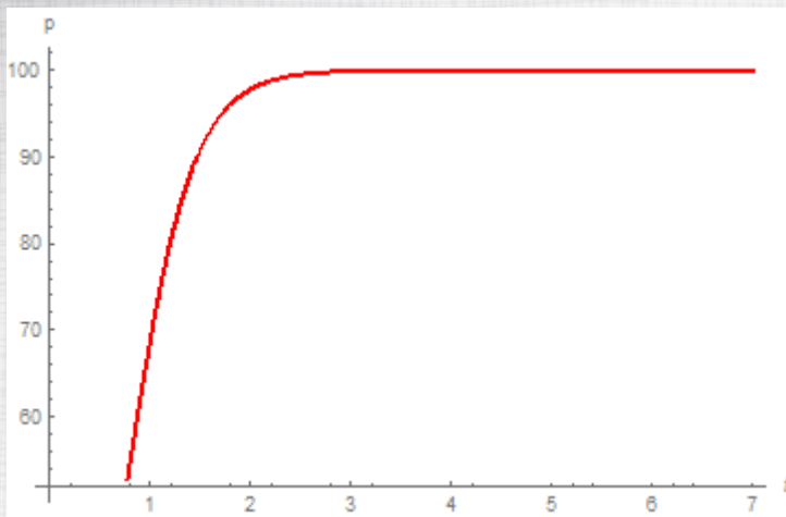
Figura 3: Población versus tiempo, problema 2.
