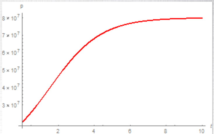
Figura 5: Gráfica del modelo logístico, problema 4.
