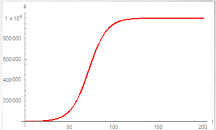
Figura 2: Capacidad de soporte, problema 1.
