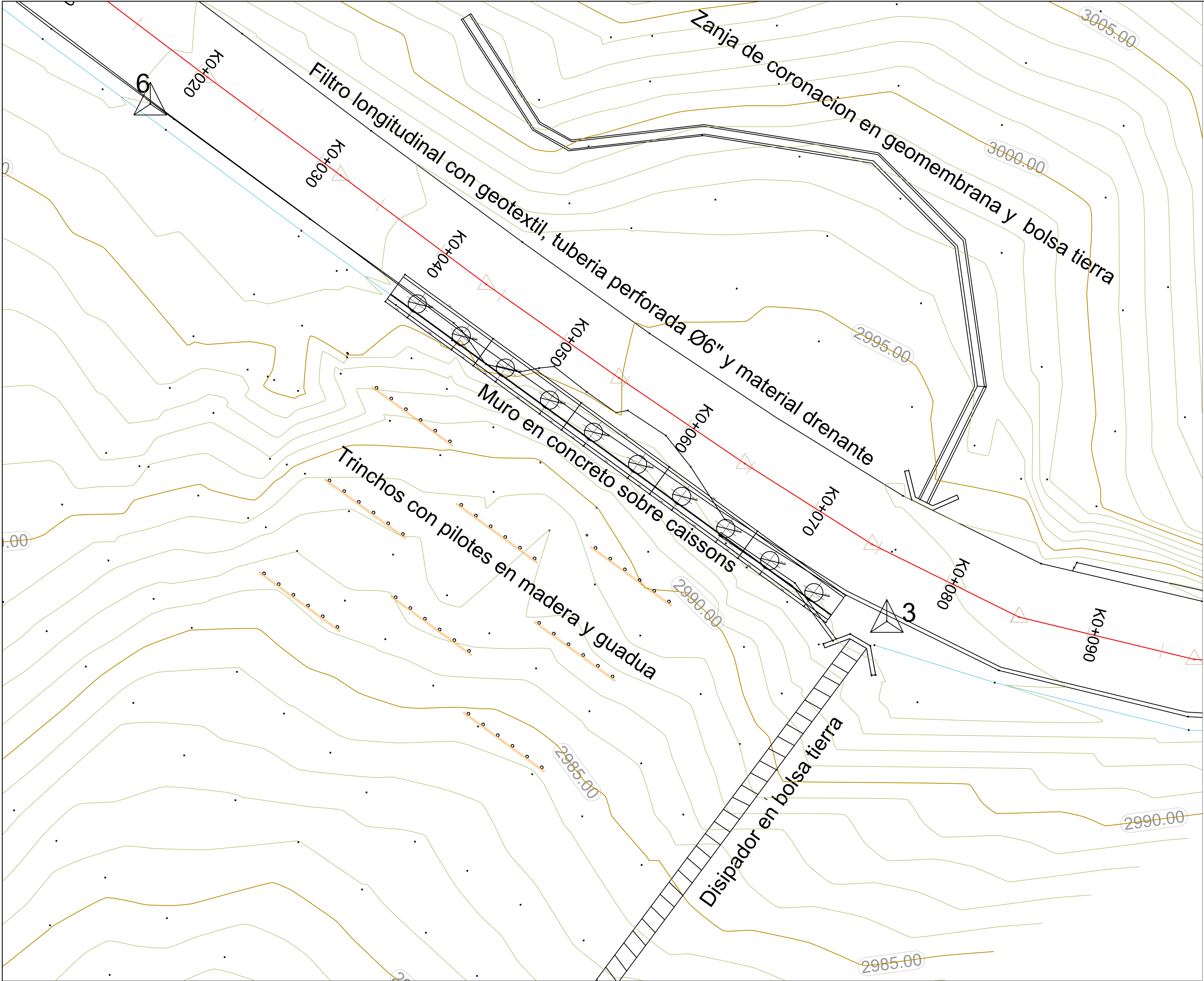
PLANTA - LOCALIZACIÓN GENERAL DE LAS OBRAS PARA SOLUCIÓN DEFINITIVA Escala 1:125
