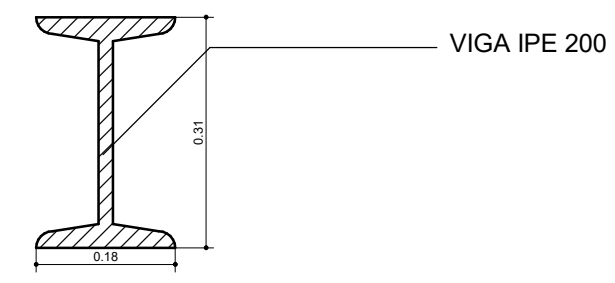
1 DETALLE VIGA IPE 200 1:10
