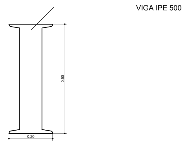
2 DETALLE VIGA IPE 500 1:10
