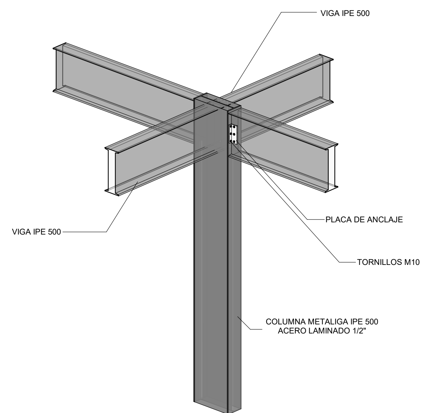
4 VISTA 3D UNIÓN VIGAS
