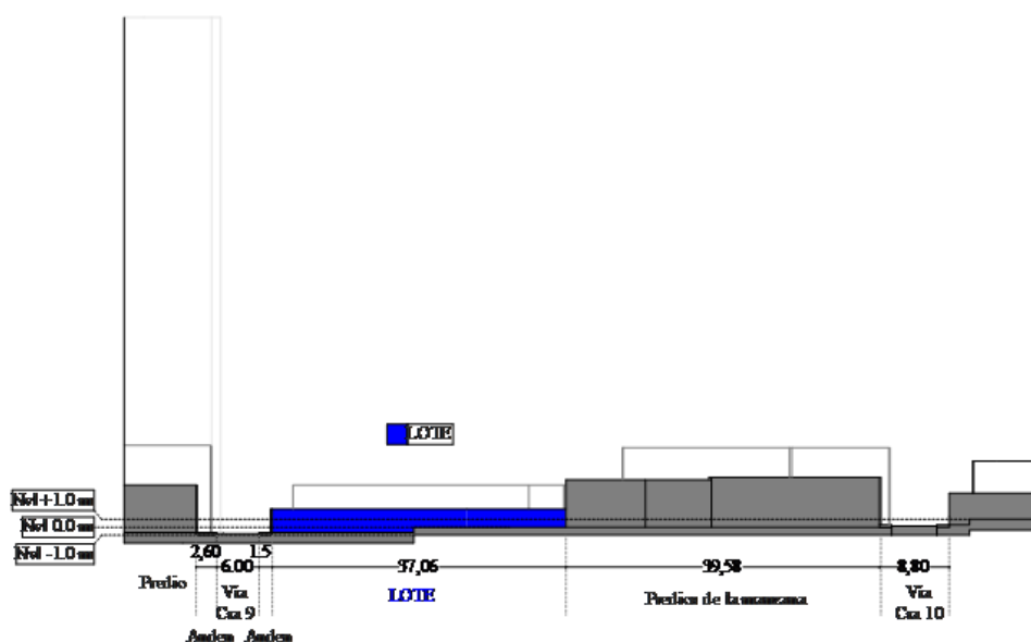
Figura 52. Sección longitudinal lote.
