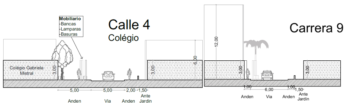
Figura 54. Perfil vial calle 4 y carrera 9.
