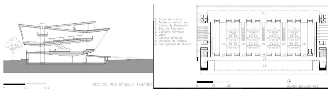
Figura 9. Sección y plano segundo piso biblioteca EPM
