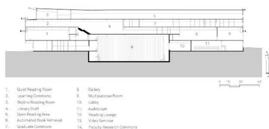
Figura 24. Sección biblioteca James Hunt.
