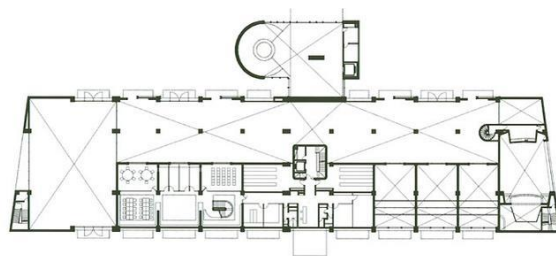
Figura 12. Plano segundo piso biblioteca el tintal. Bogotá.
