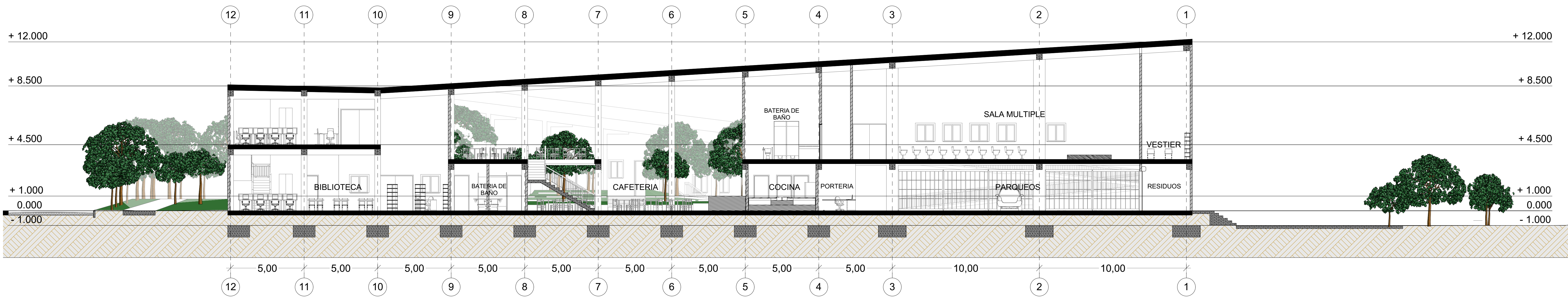
SECCIÓN D - D' ESC: 1:125
