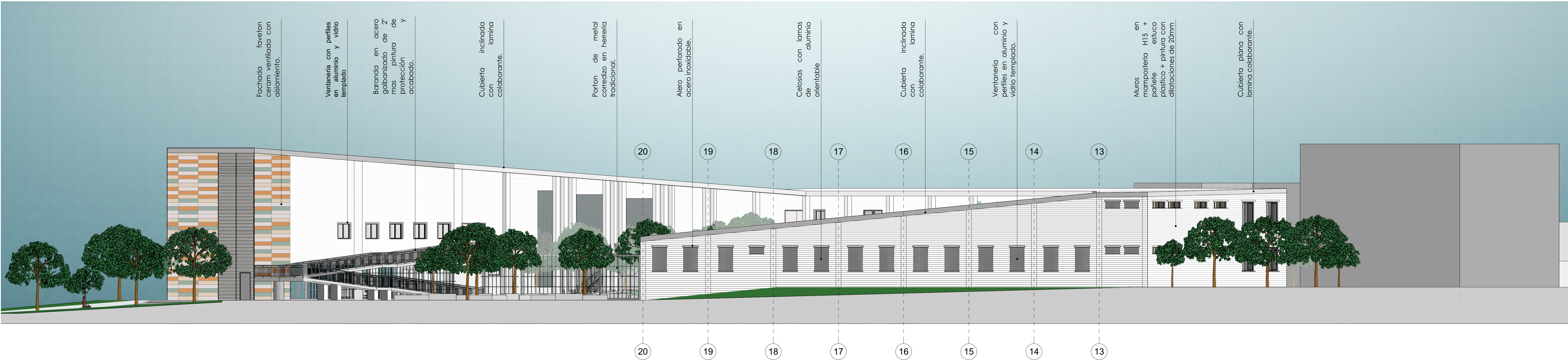
FACHADA SUR-OCCIDENTE ESC: 1:125
