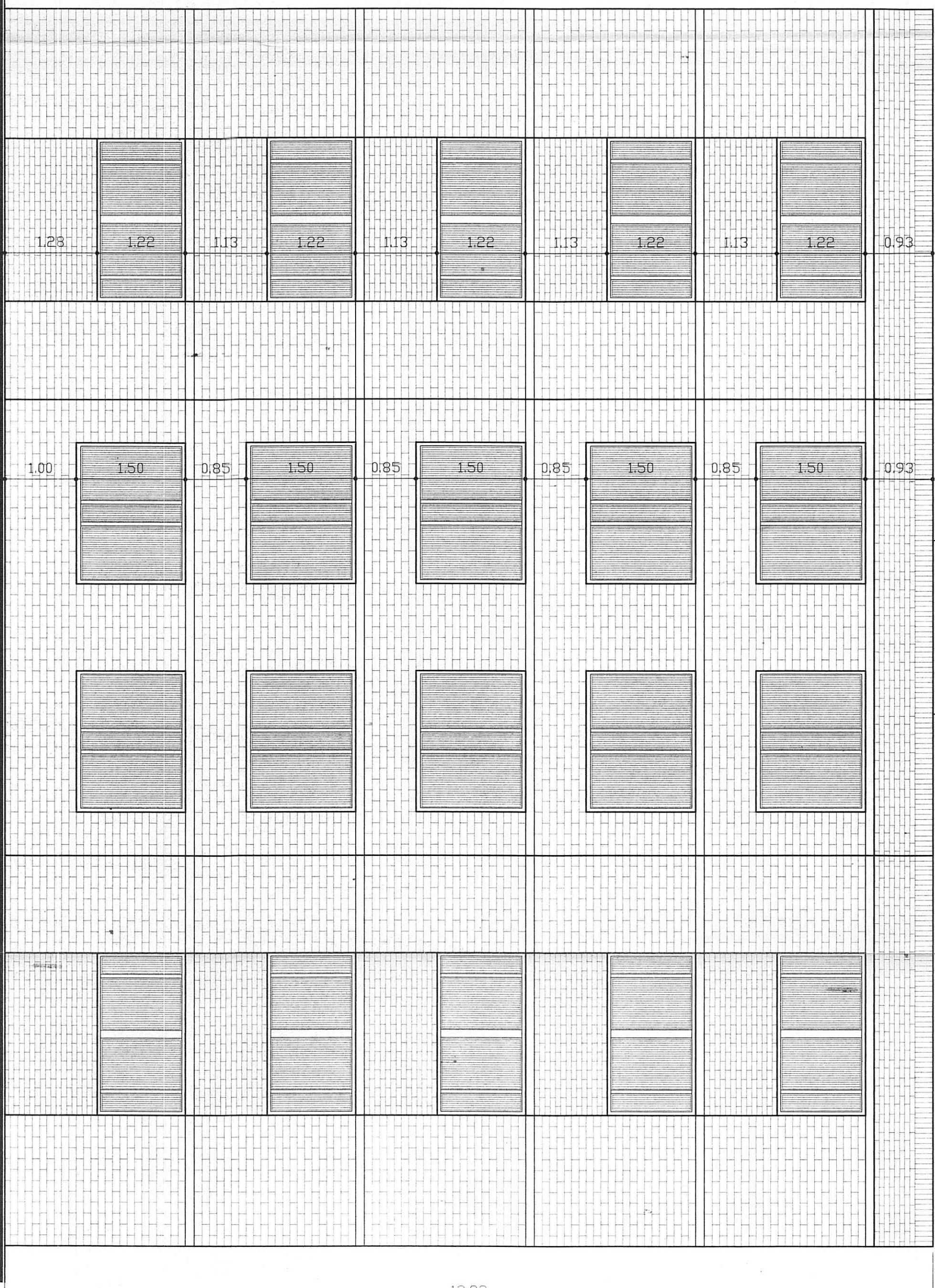
FACHADA POSTERIOR Esc. 1 : 50
