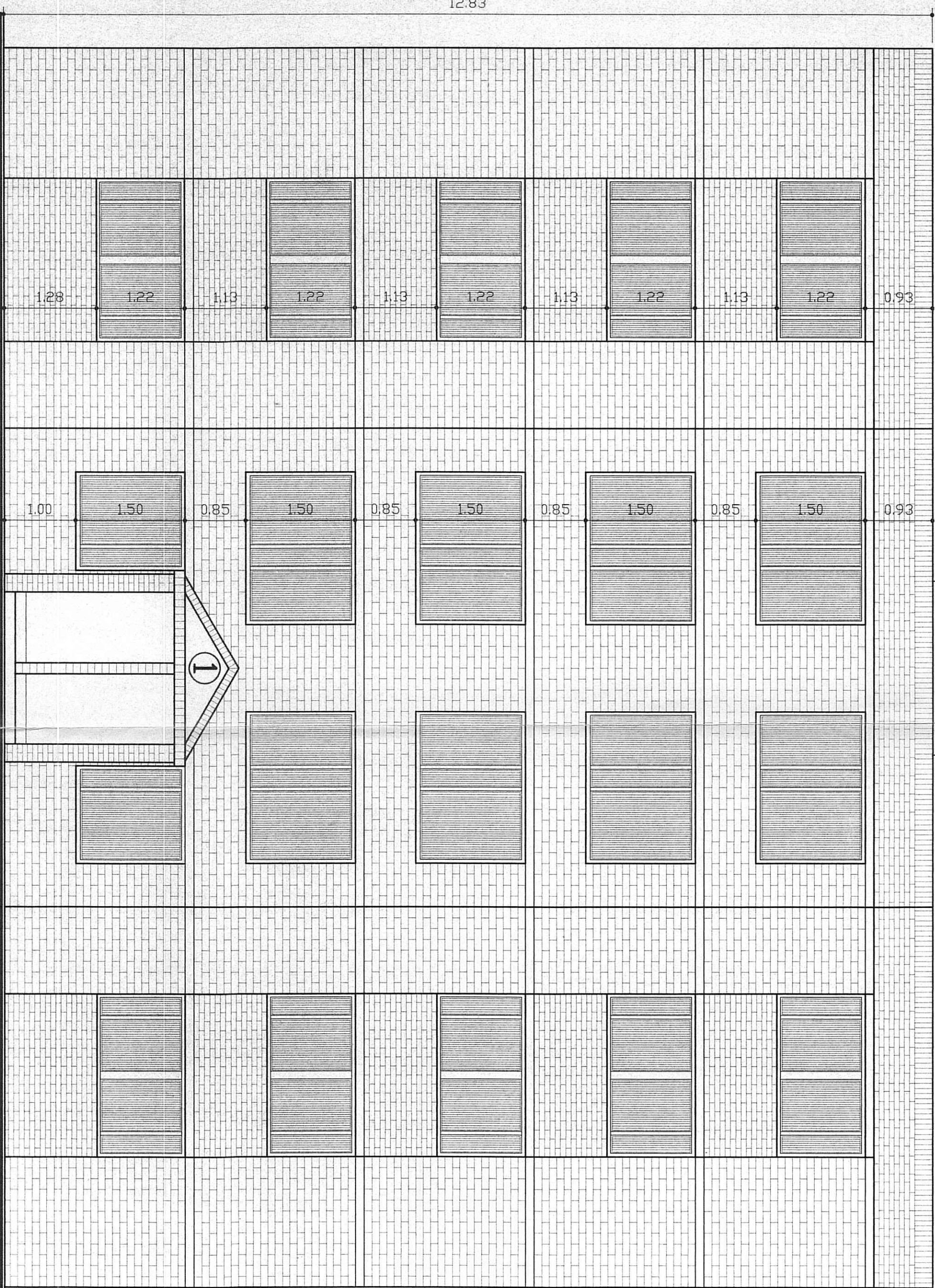
FACHADA PRINCIPAL Esc. 1 : 50
