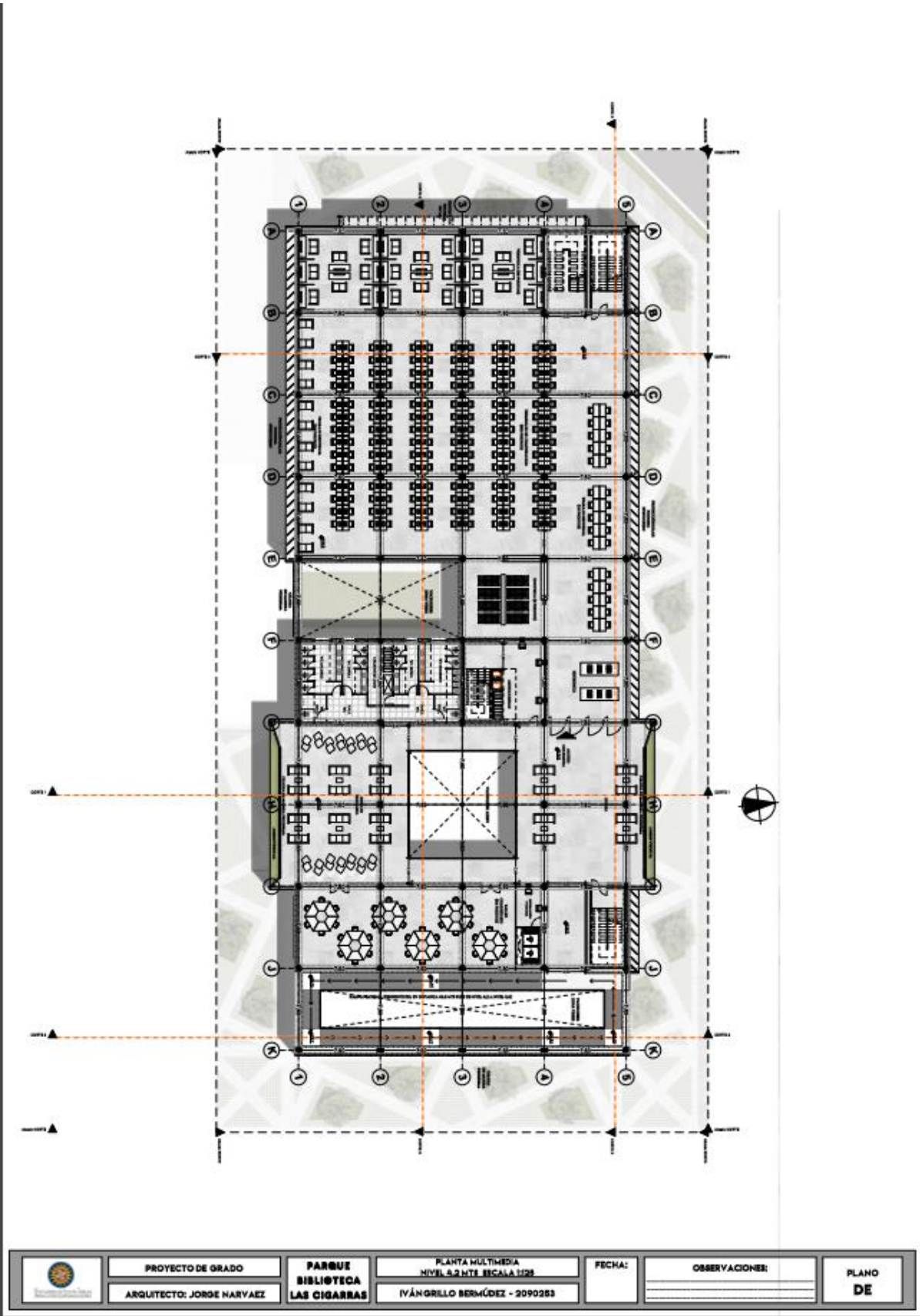
Figura 49. Planta Multimedia
