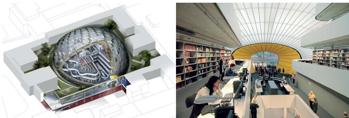
Figura 10. Biblioteca Universidad Filológica, Norman Foster, Fuente http://es.wikiarquitectura.com/index.php/Archivo:Blib_Filolog_Berlin_11.jpg
