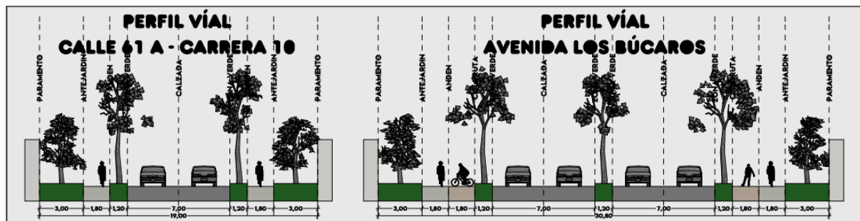
Figura 39. Perfiles Viales Propuestos.
