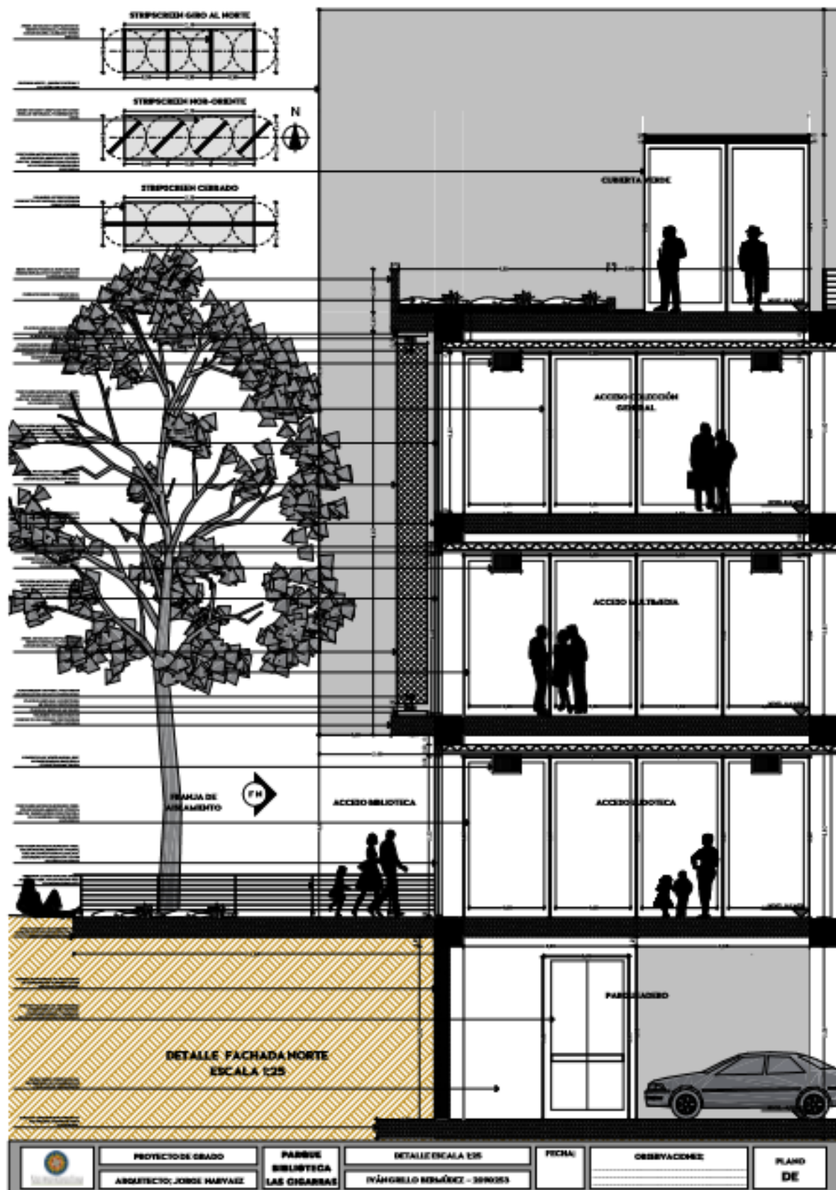
Figura 54. Detalle Fachada Norte
