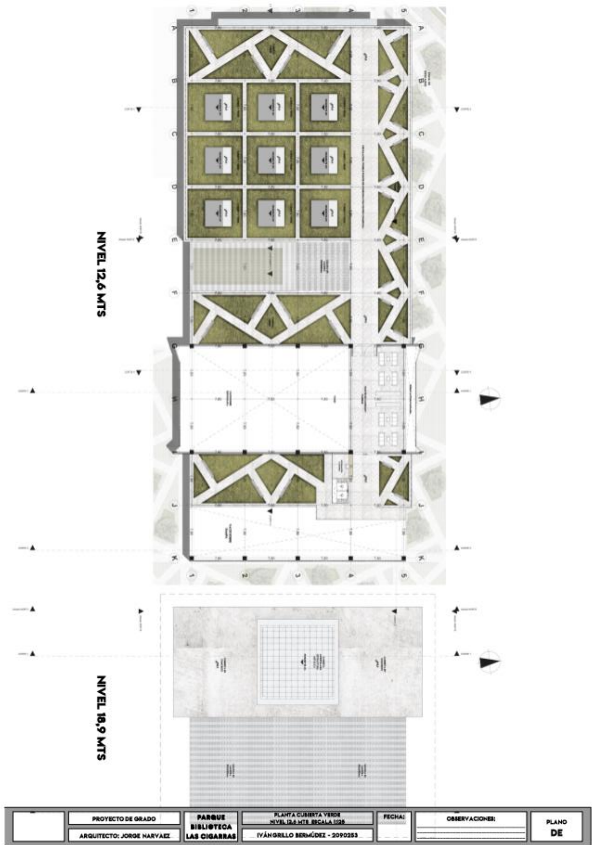
Figura 51. Planta Cubierta Verde
