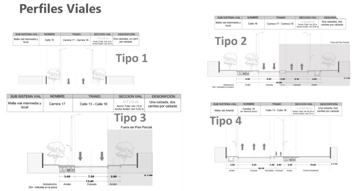
Figura 17. Perfiles Viales Propuestos.
