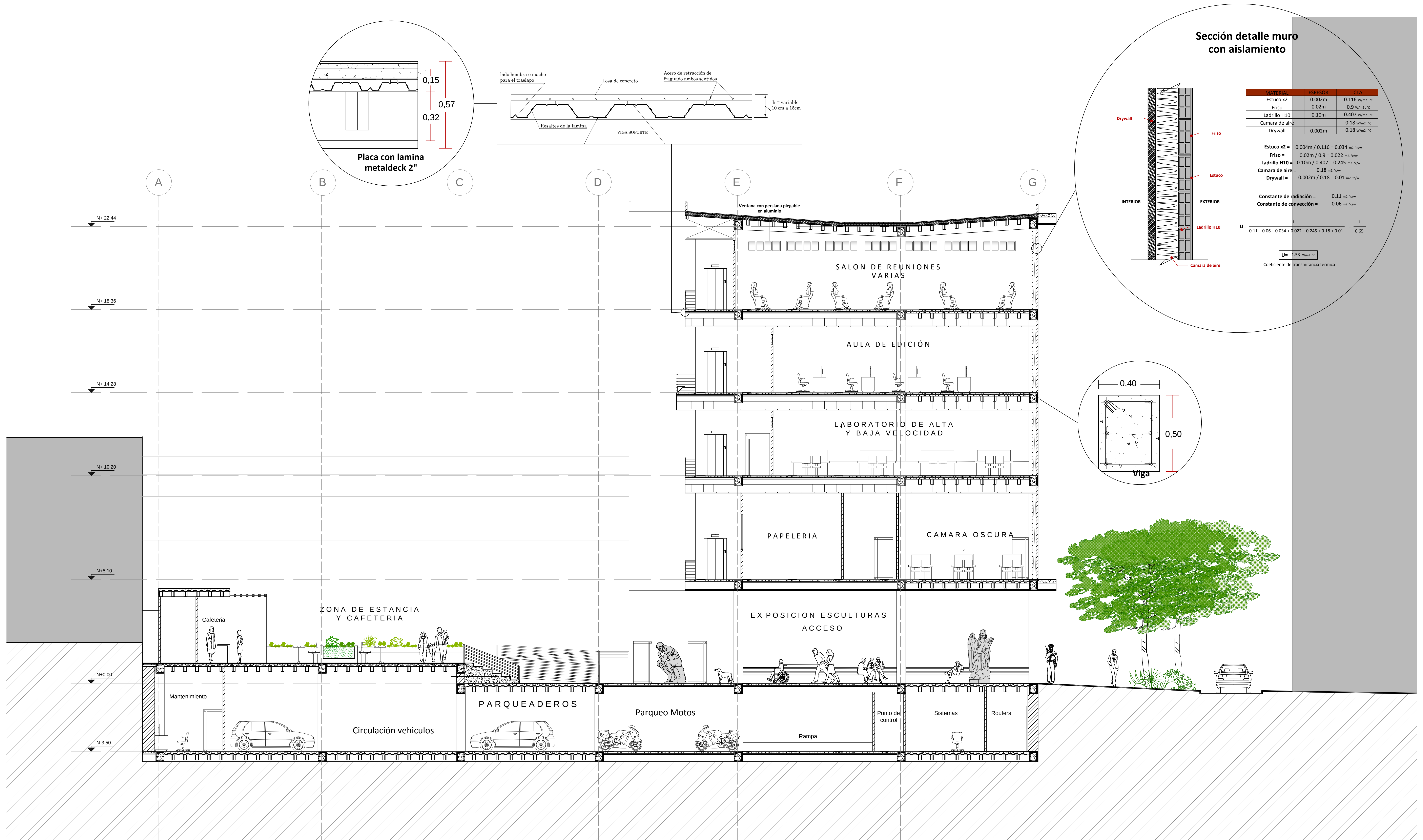
CORTE A-A' Esc: 1_75
