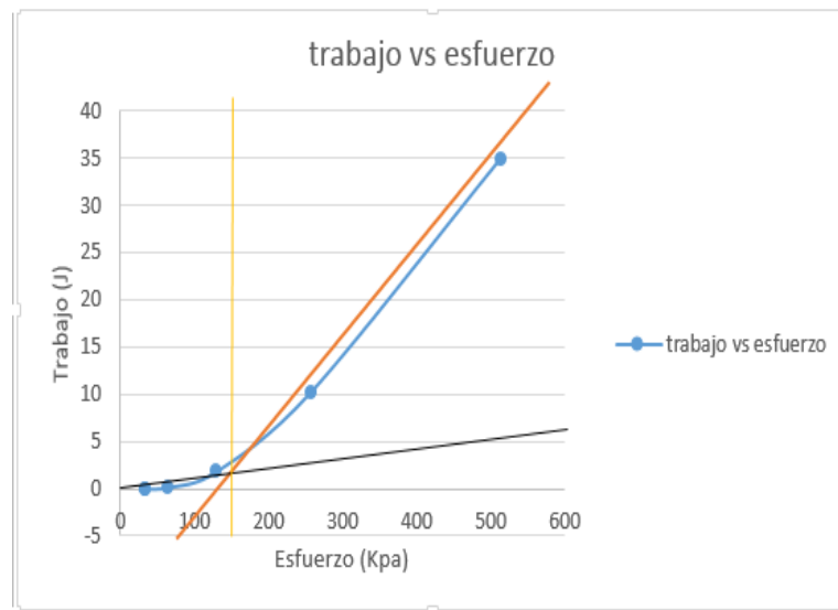
Figura 56. Carga de preconsolidacion Sondeo 1 Muestra3
