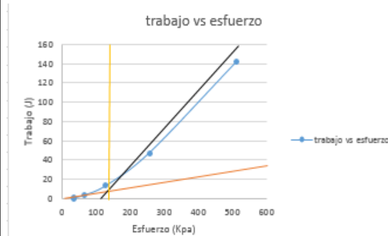
Figura 64. Carga de preconsolidacion
