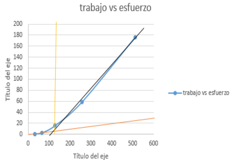
Figura 58. Carga de preconsolidacion sondeo 1 muestra 17
