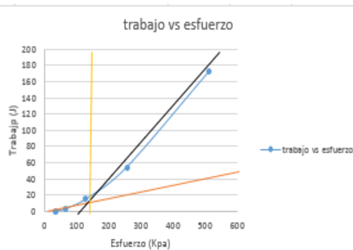
Figura 63. Carga de preconsolidacion, sondeo, muestra 23
