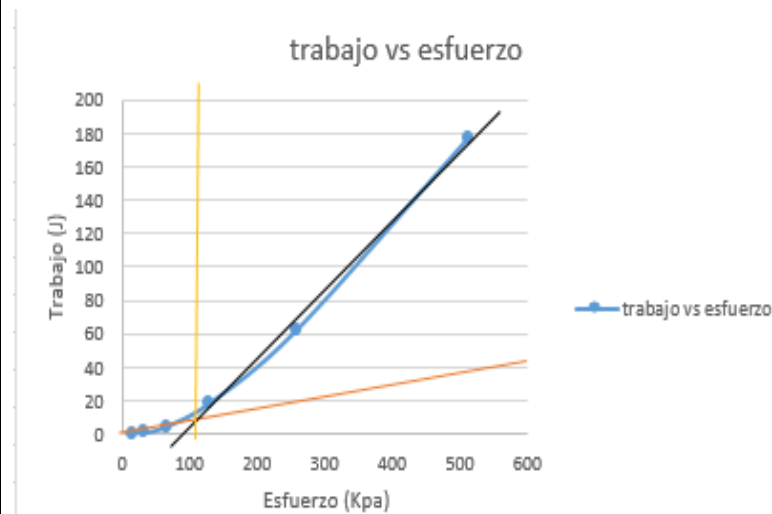
Figura 57. Carga de preconsolidacion Sondeo 1 muestra 11
