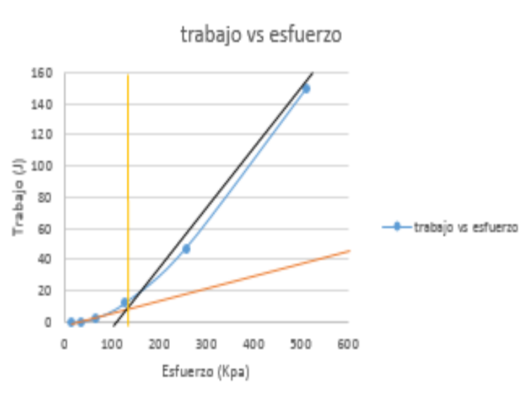
Figura 60. Carga de preconsolidacion, sondeo 1 muestra 29
