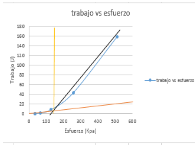
Figura 59. Carga de preconsolidacion, sondeo 1 muestra 25
