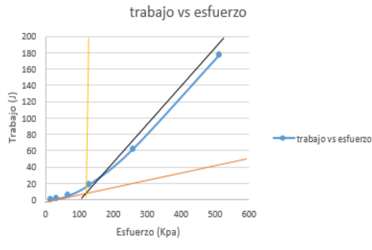
Figura 61. Carga de preconsolidacion, sondeo 2 muestra 11
