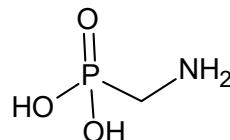
Figura 2. Ácido aminometilfosfónico (AMPA)
