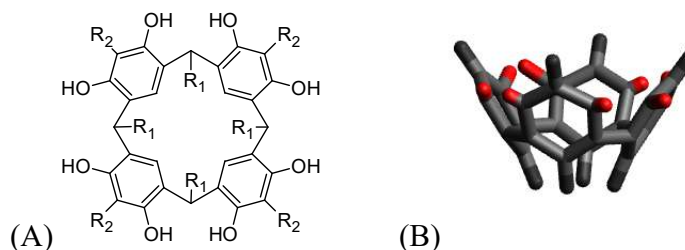
Figura 4. Resorcinarenos propuestos en el presente estudio. Na 4 MeRA R 1 =-CH 3 , R 2 =CH 2 SO 3 Na; Na 4 EtRA R 1 =-CH 2 CH 3 , R 2 = CH 2 SO 3 Na; Na 4 PrRA R 1 =-CH 2 CH 2 CH 3 , R 2 = CH 2 SO 3 Na; Na 4 SRA R 1 =-CH 2 CH 2 SCH 3 , R 2 = CH 2 SO 3 Na; Na 4 ESRA R 1 =-CH 2 CH 2 SO 3 Na, R 2 =H Estructura típica en forma de copa de Resorcinareno (B)
