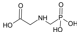
Figura 1. Molécula del N-(fosfonometil)glicina (Glifosato)
