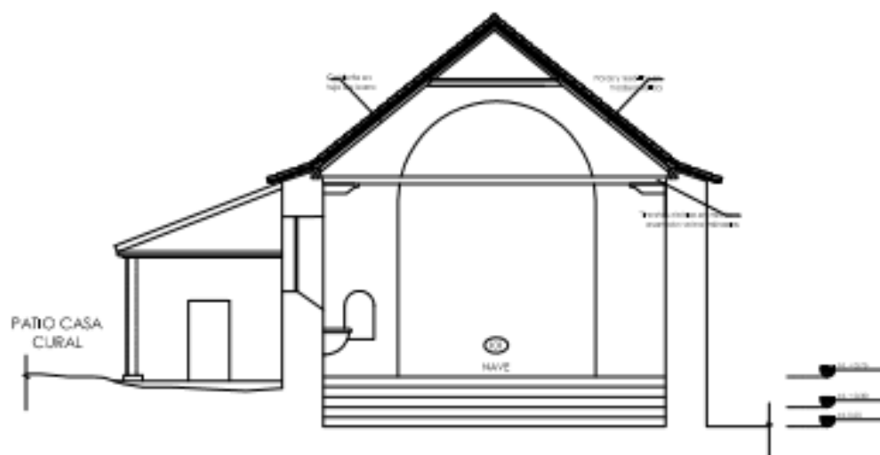
Plano 14: Corte Transversal. Templo Doctrinero
