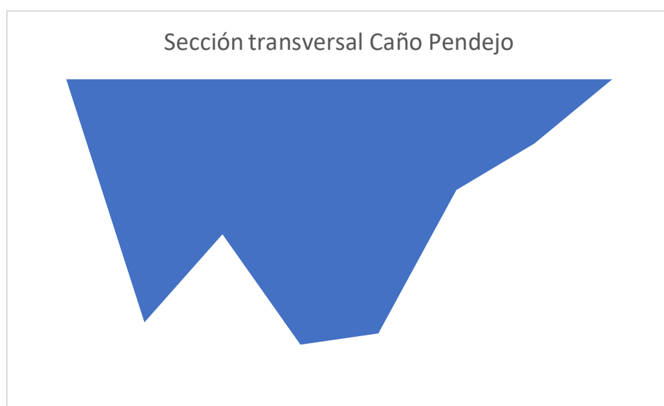
Ilustración 1. Sección transversal caño pendejo, Fuente: autores.
