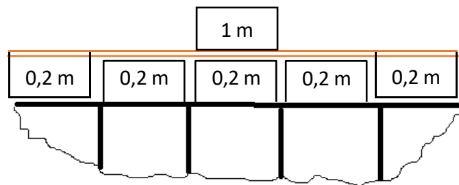
Ilustración 1. Representación del procedimiento de batimetría, Fuente: autores.
