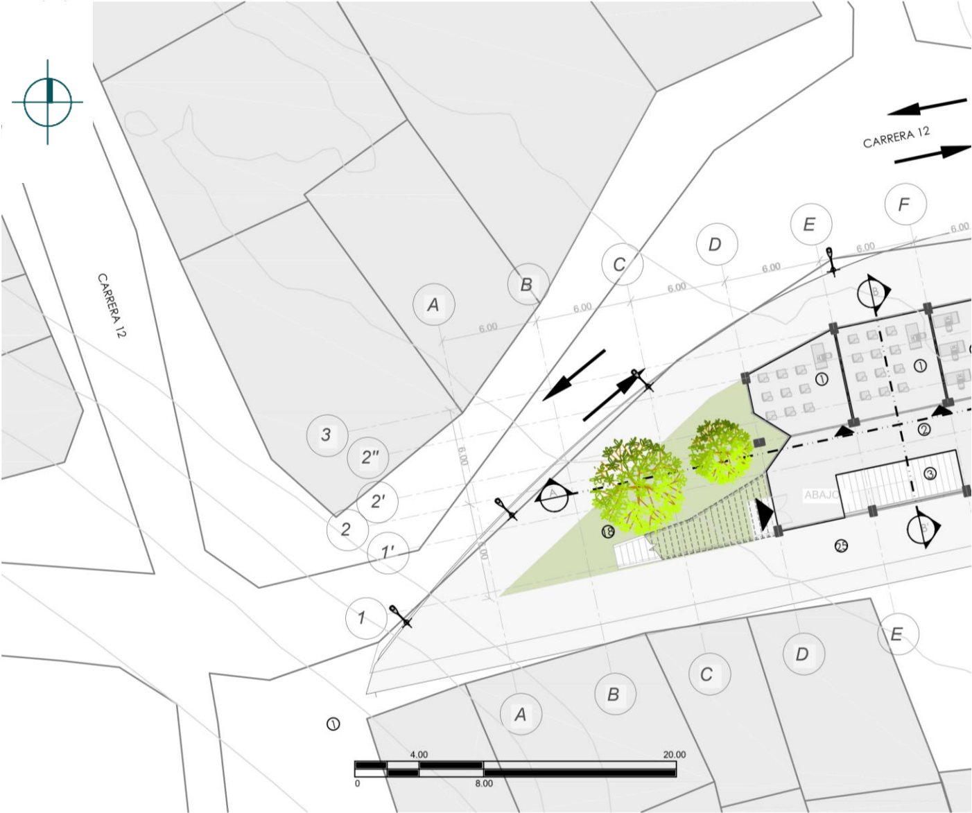
Figura 55- Planimetría- Elaboración propia
