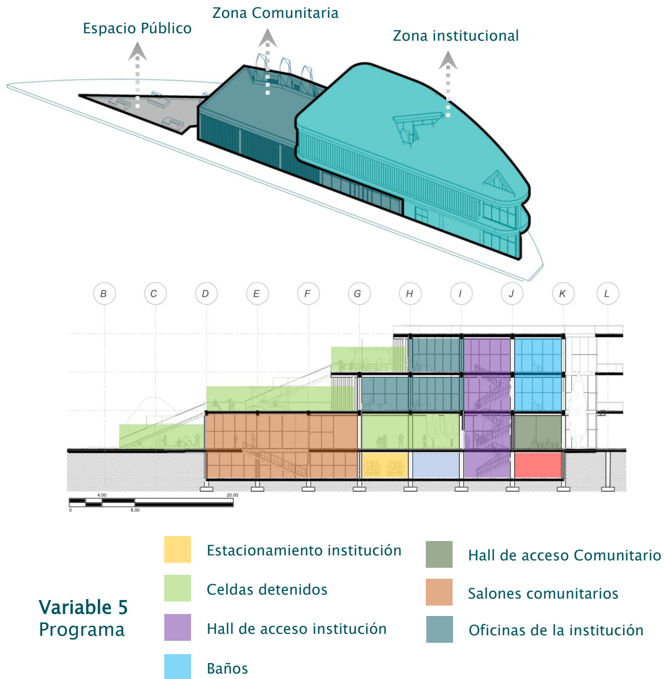
Figura 51 – Esquema estrategias – Elaboración propia
