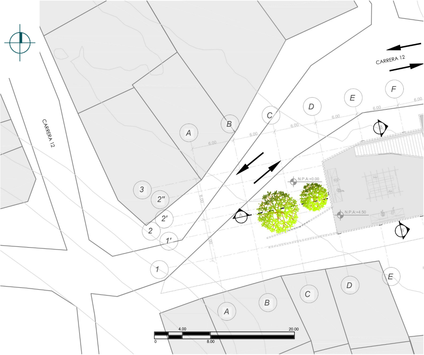
Figura 58- Planimetría- Elaboración propia
