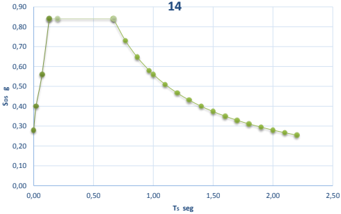
espectro elástico de Aceleraciones de diseño CCP 14
