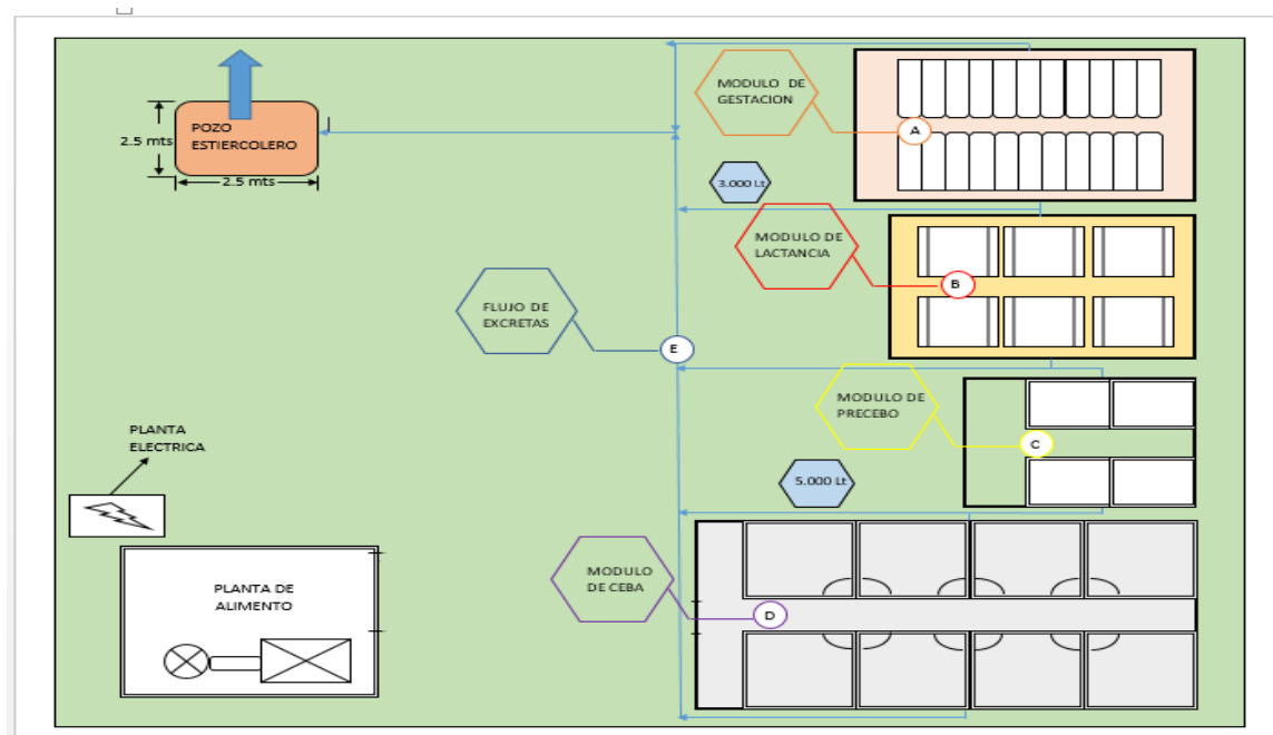
Figura 18. Esquema de distribución de planta. (QUALITY PORK S.A.S, 2018).
