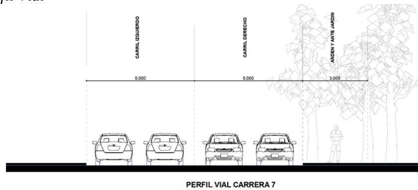
Figura 34. Perfil Vial
