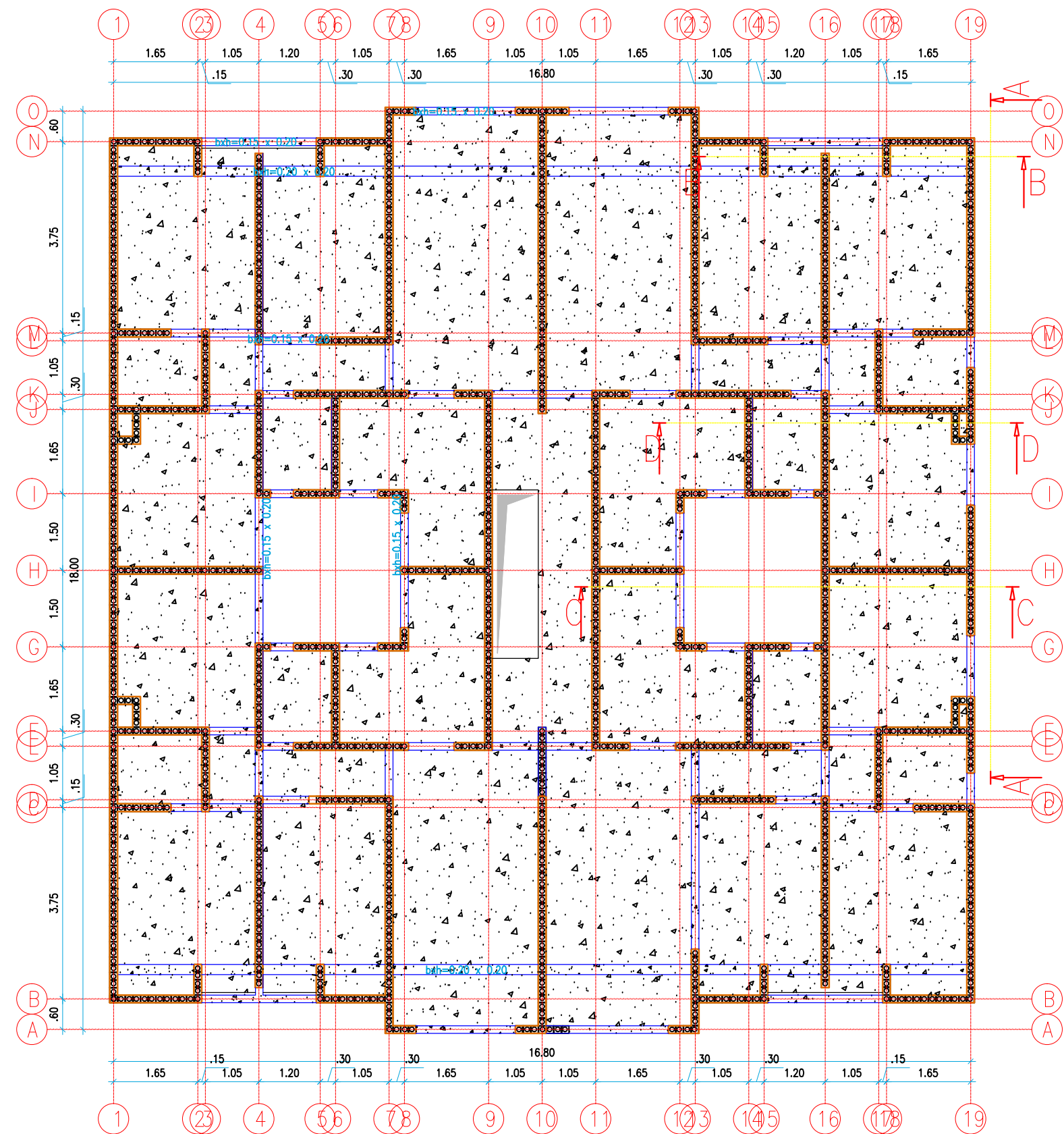
Cubierto (+12.00 m)
