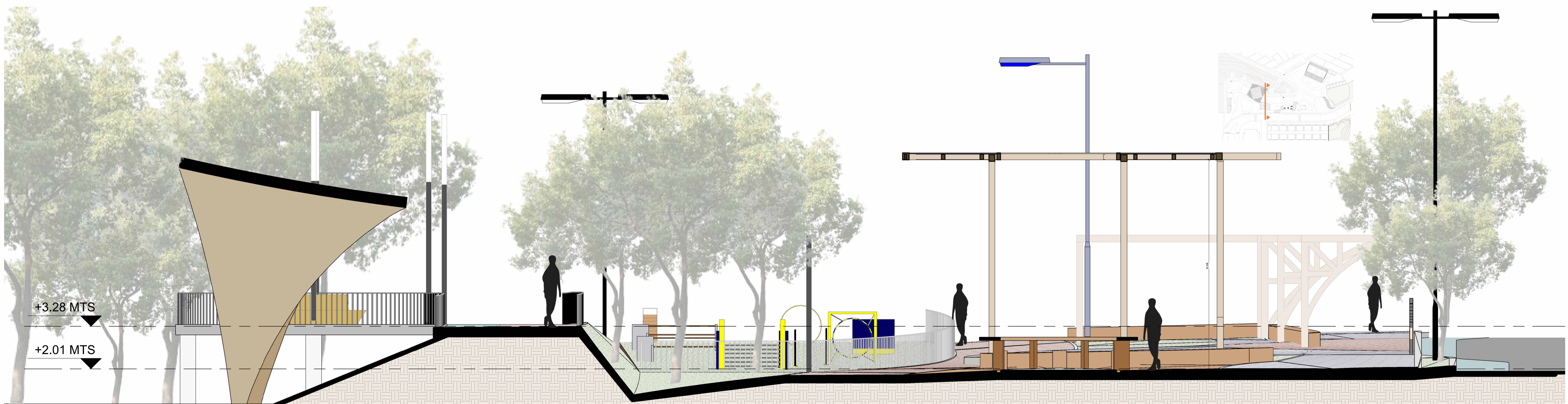
CORTE C-C' ESC. 1.100
