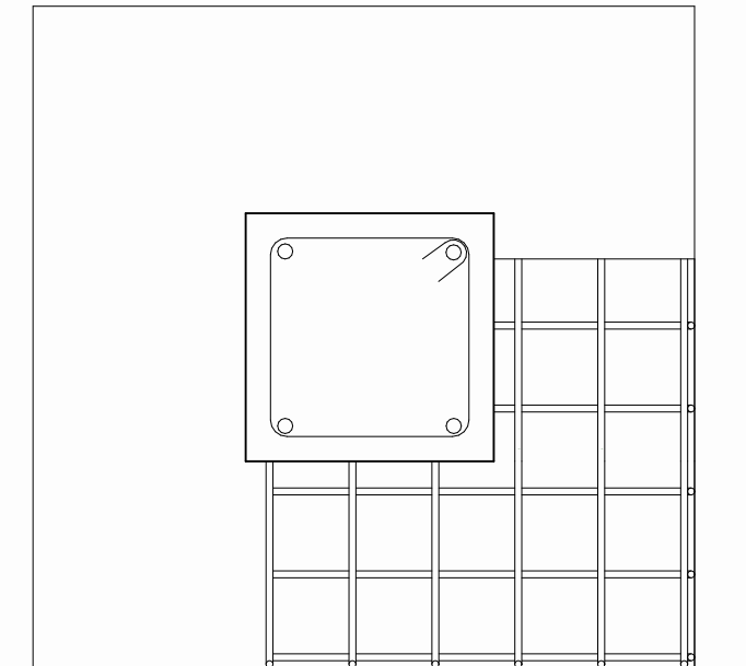
Zapata Aislada-Tipo1 Parilla armada con var. 1/2" cada 10 cms en ambos sentidos
