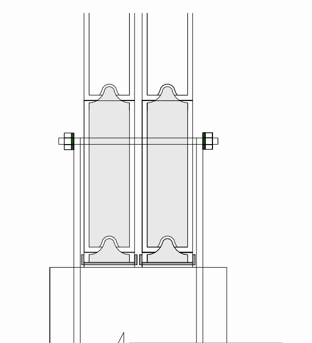
Detalle constructivo Anclaje bambu Perno externo
