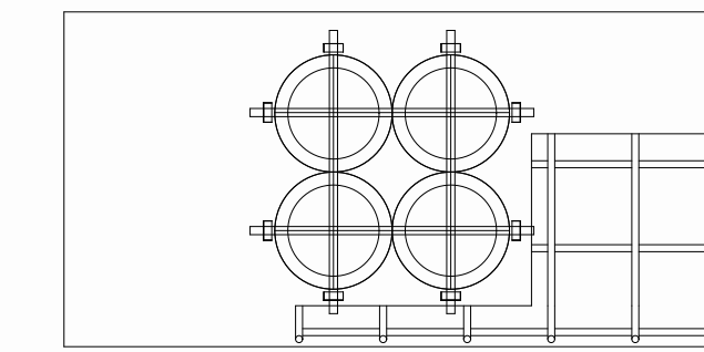
Zapata Aislada-Tipo2 Parilla armada con var. 1/2" cada 10 cms
