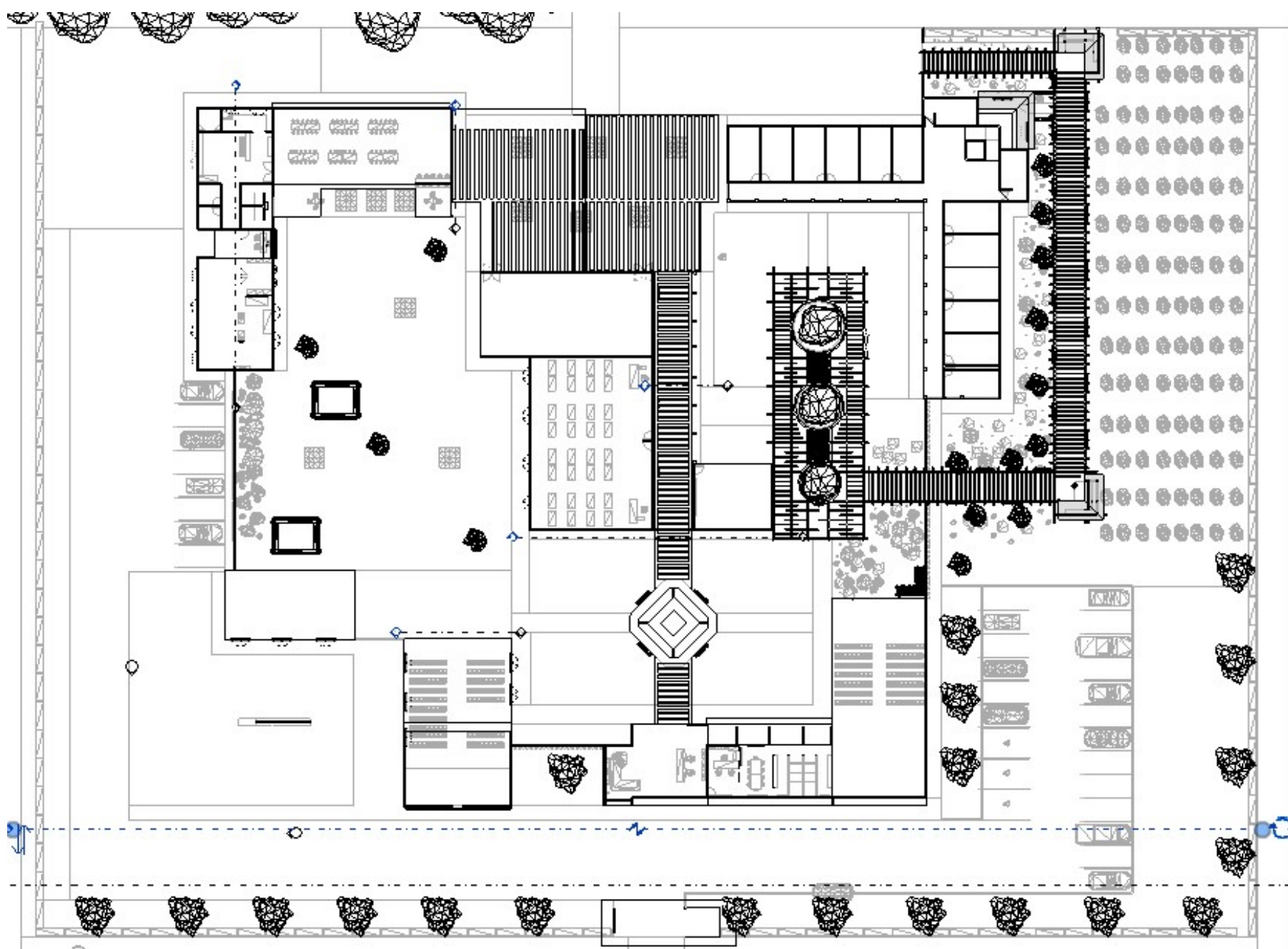
Planta 2do Piso - Autoría Propia
