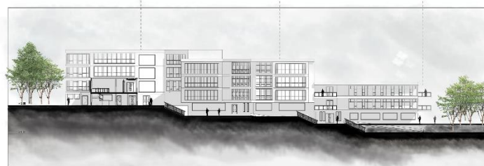
CORTE DORMITORIOS NIÑOS DE 6 A 12 AÑOS 1:200
