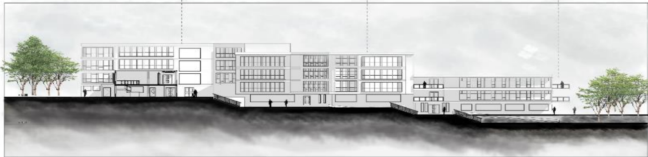
FACHADA PRIVADO EDIFICIO DE DORMITORIOS 1:200
