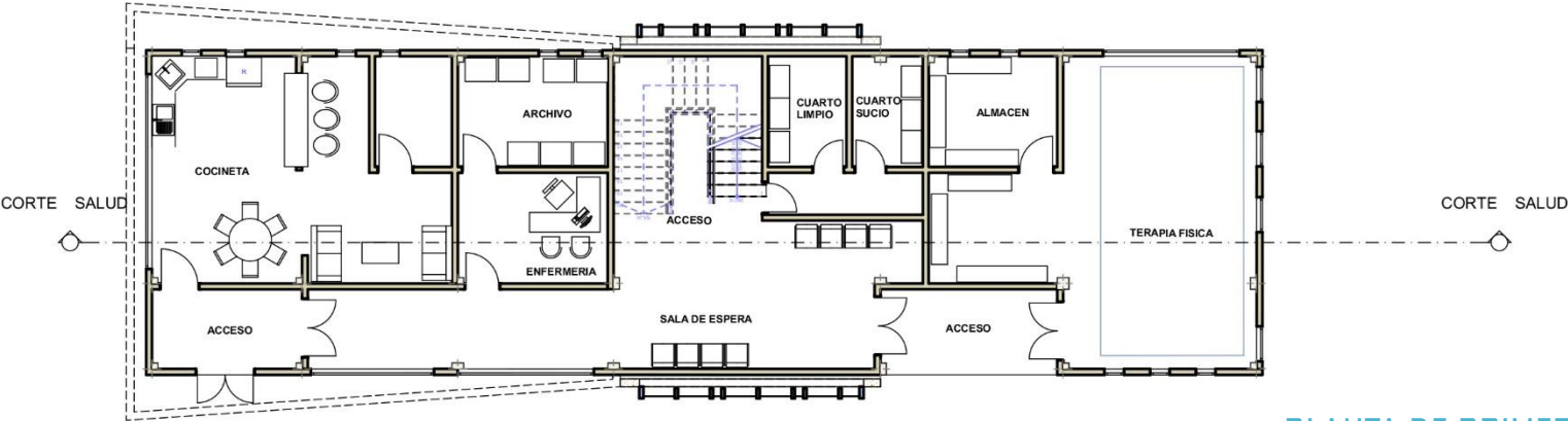
PLANTA DE PRIMER PISO
