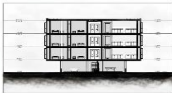
CORTE DORMITORIOS ADOLESCENTES 13 A 17 AÑOS 1:200
