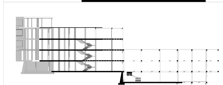
CORTE ESTRUCTURAL DORMITORIOS
