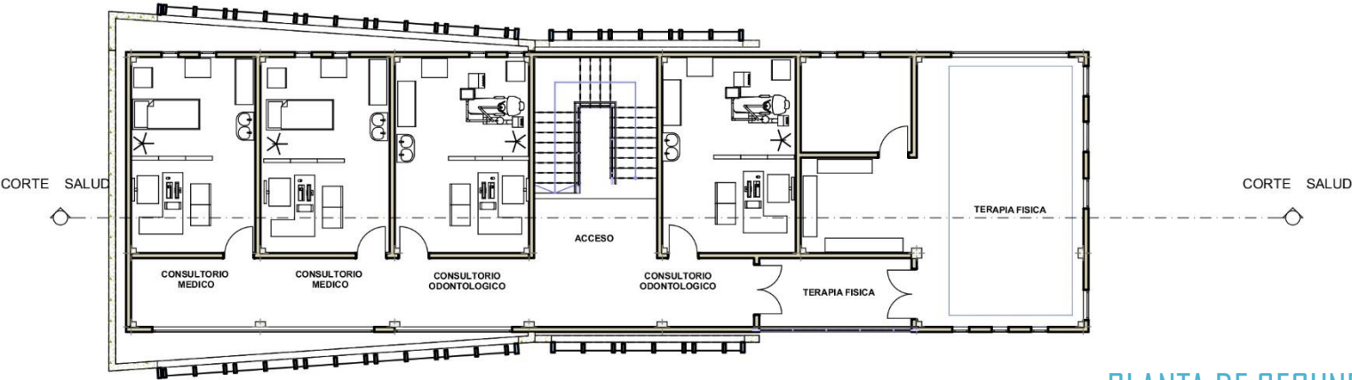
PLANTA DE SEGUNDO PISO
