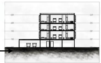
CORTE DORMITORIOS NIÑOS DE 6 A 12 AÑOS 1:200
