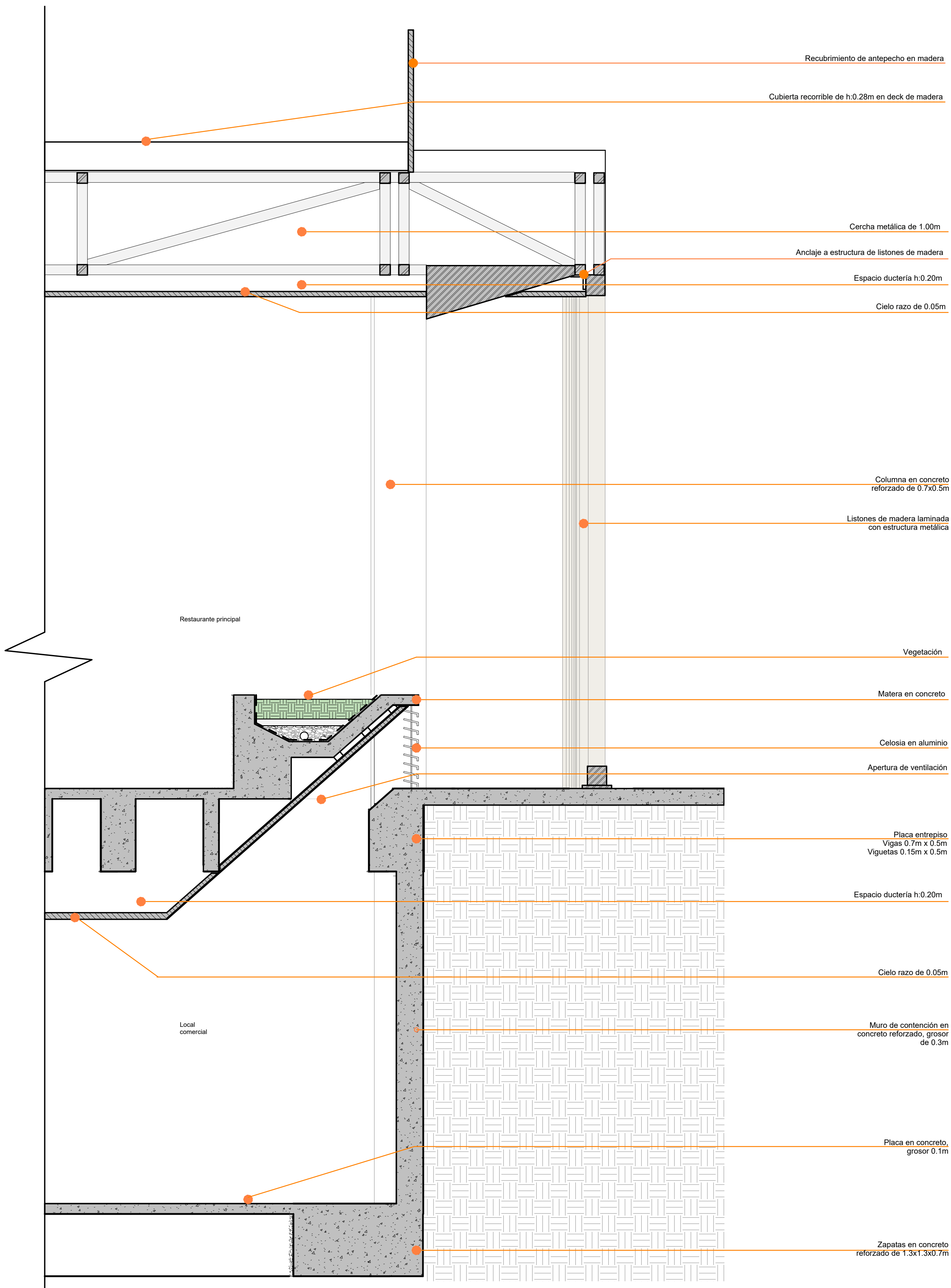
DETALLE CORTE FACHADA 2 ESC 1:25
