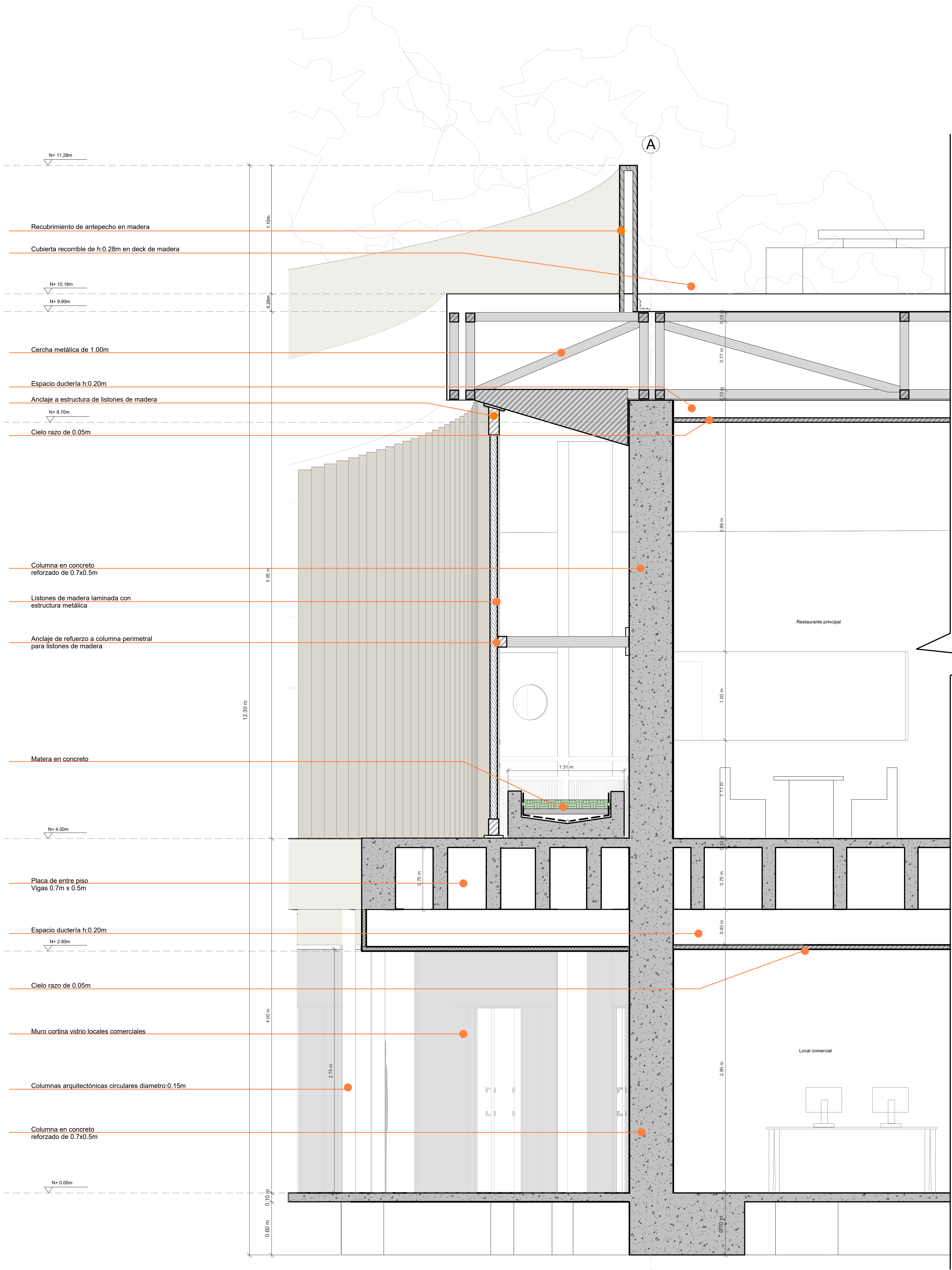
DETALLE CORTE FACHADA ESC 1:25
