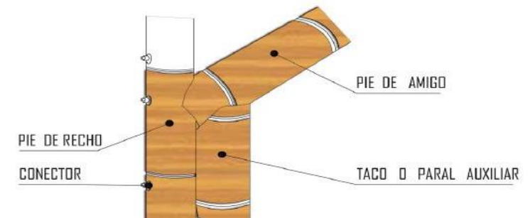
DETALLE DE UNION DE PIE DERECHO
