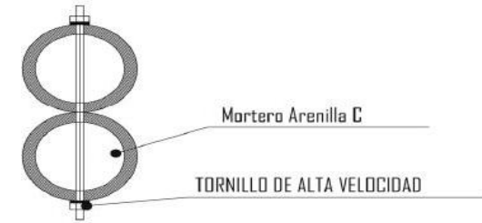
DETALLE DE TRABE DE BAMBU
