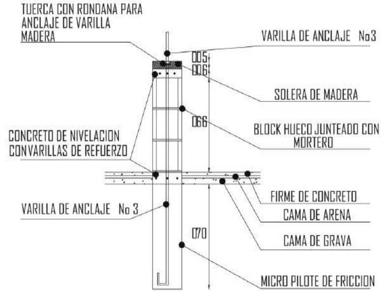
DETALLE DE CIMENTACION
