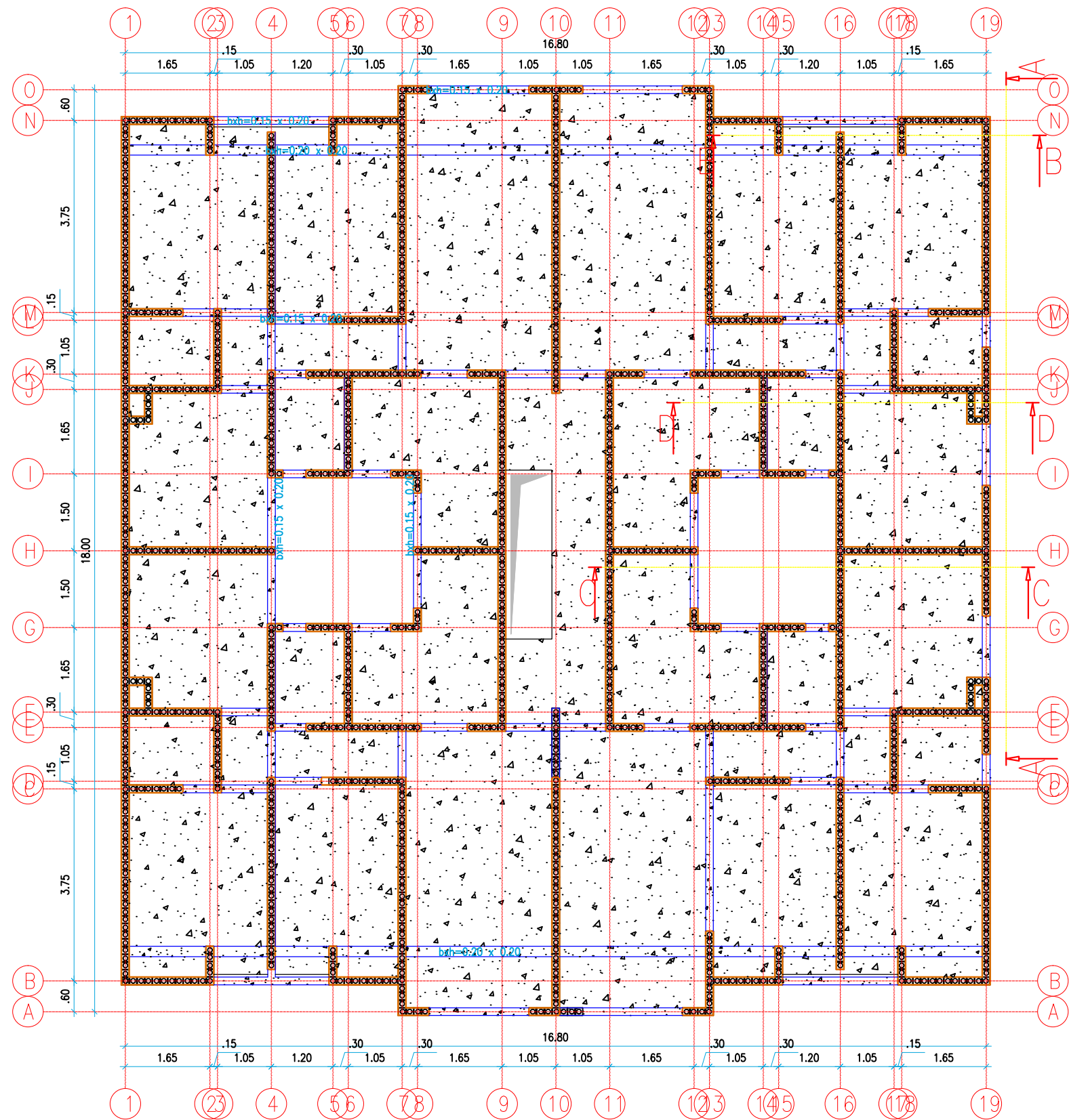
Cubierta (+12.00 m)
