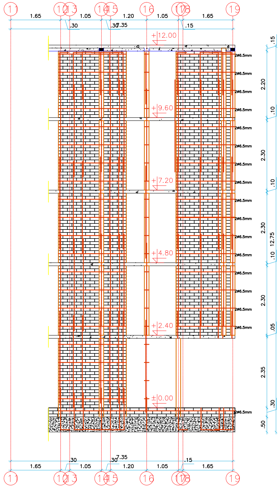
CORTE — D — D
