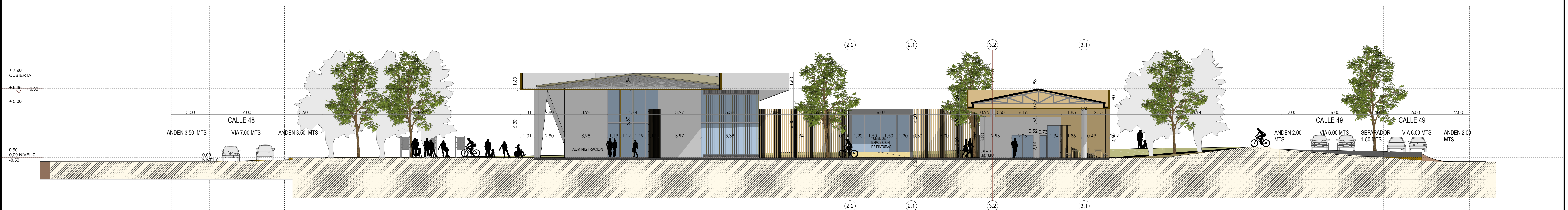
CORTE 5 ESC_1:150
