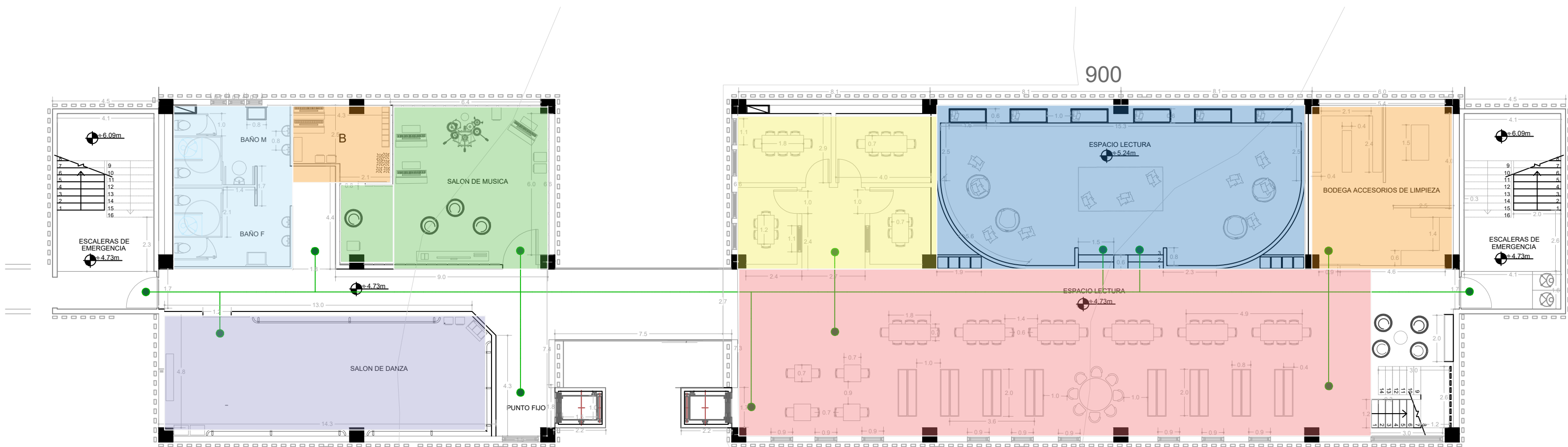
A17 PLANTA TALLER Y BIBLIOTECA SEGUNDO PISO ESC 1:150
