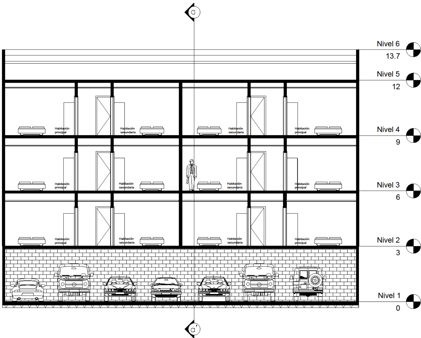
Corte b-b'
