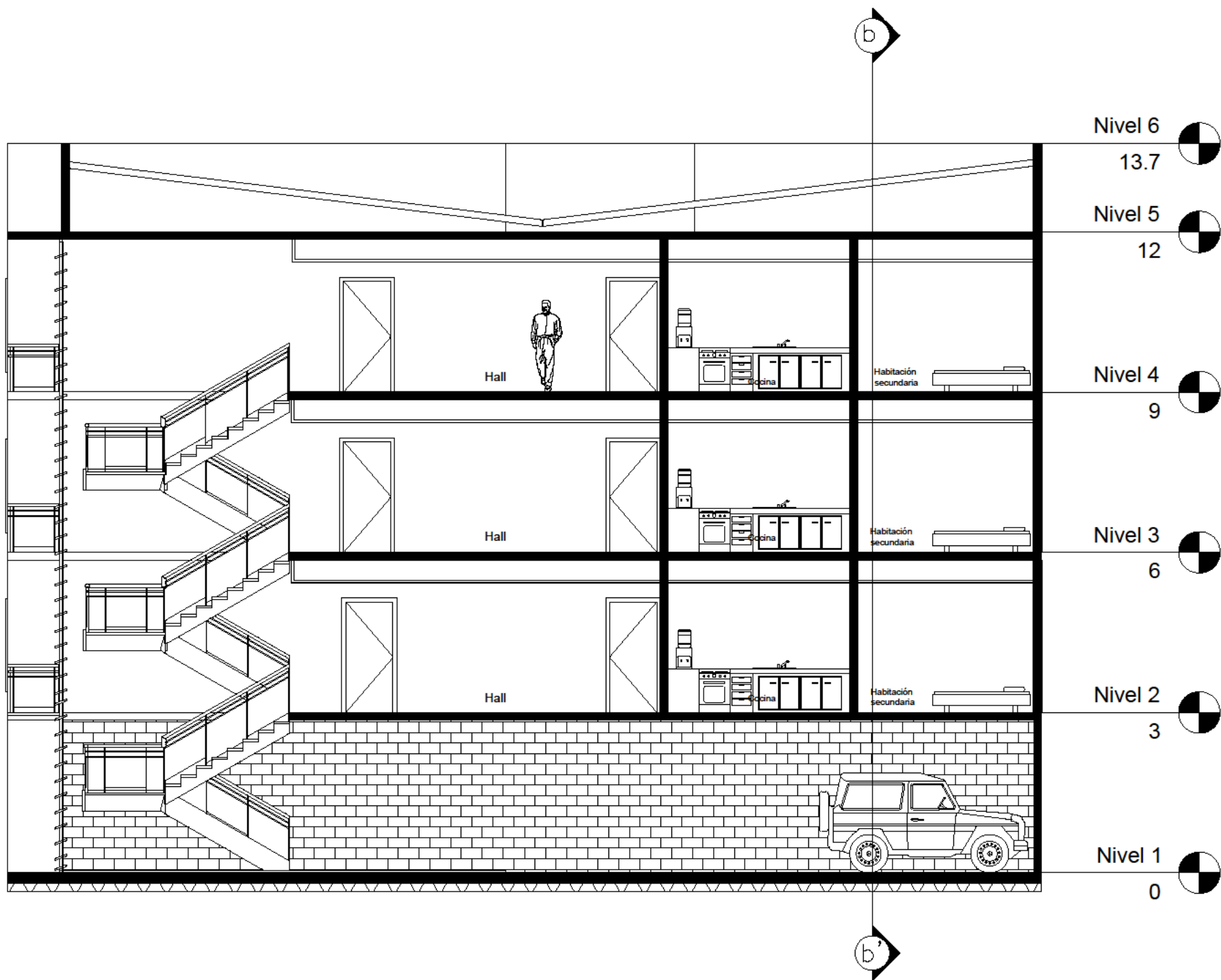
Corte a-a'
