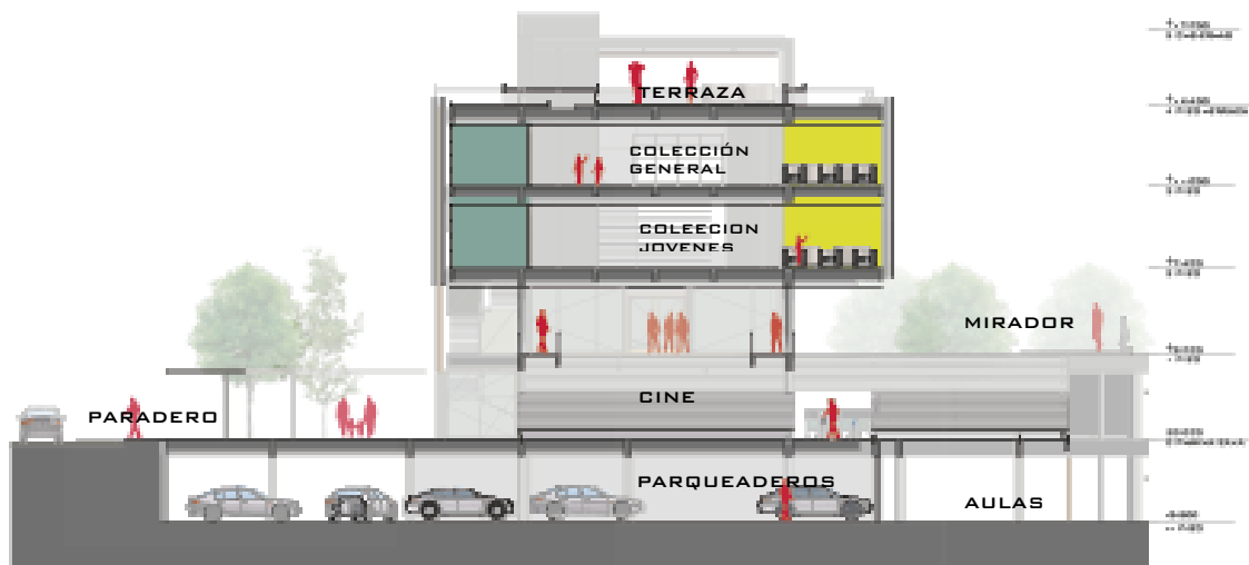
CORTE B-B ESC: REPRESENTATIVA
